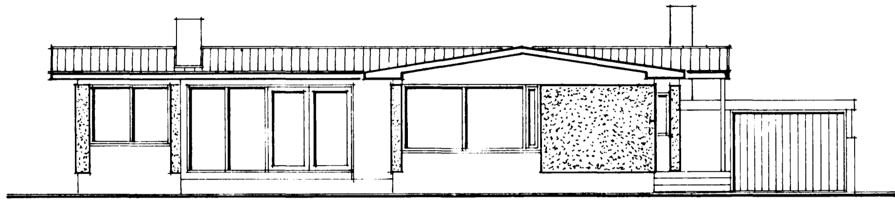
SUÐUR M.1:100
