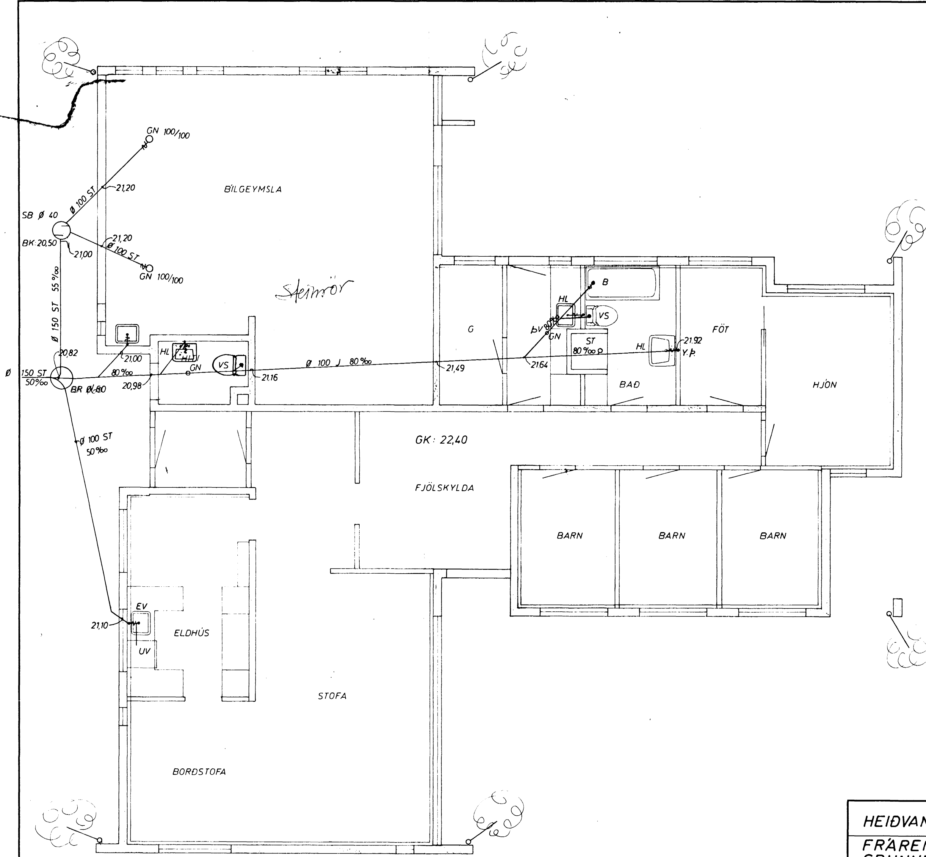
GRUNNMYND 1:50
