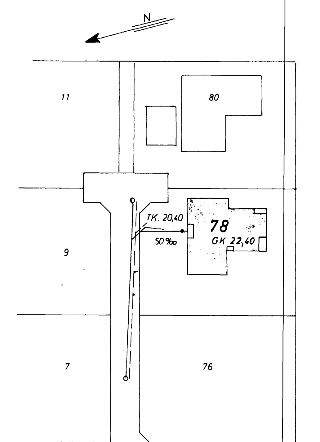
HEIÐVANGUR AFSTADA 1:500
