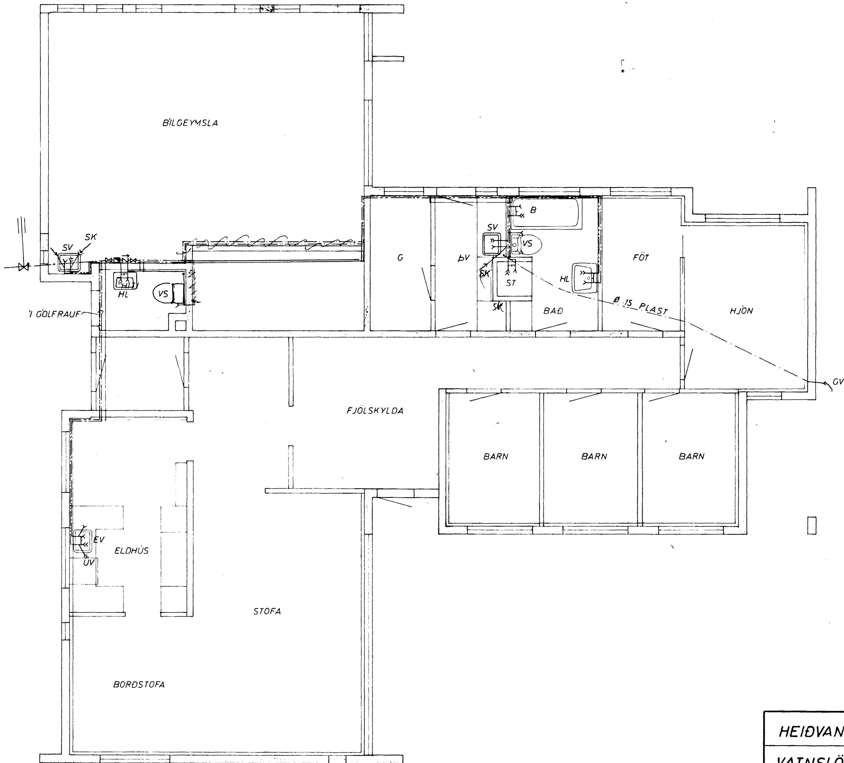
GRUNNMYND 1:50
