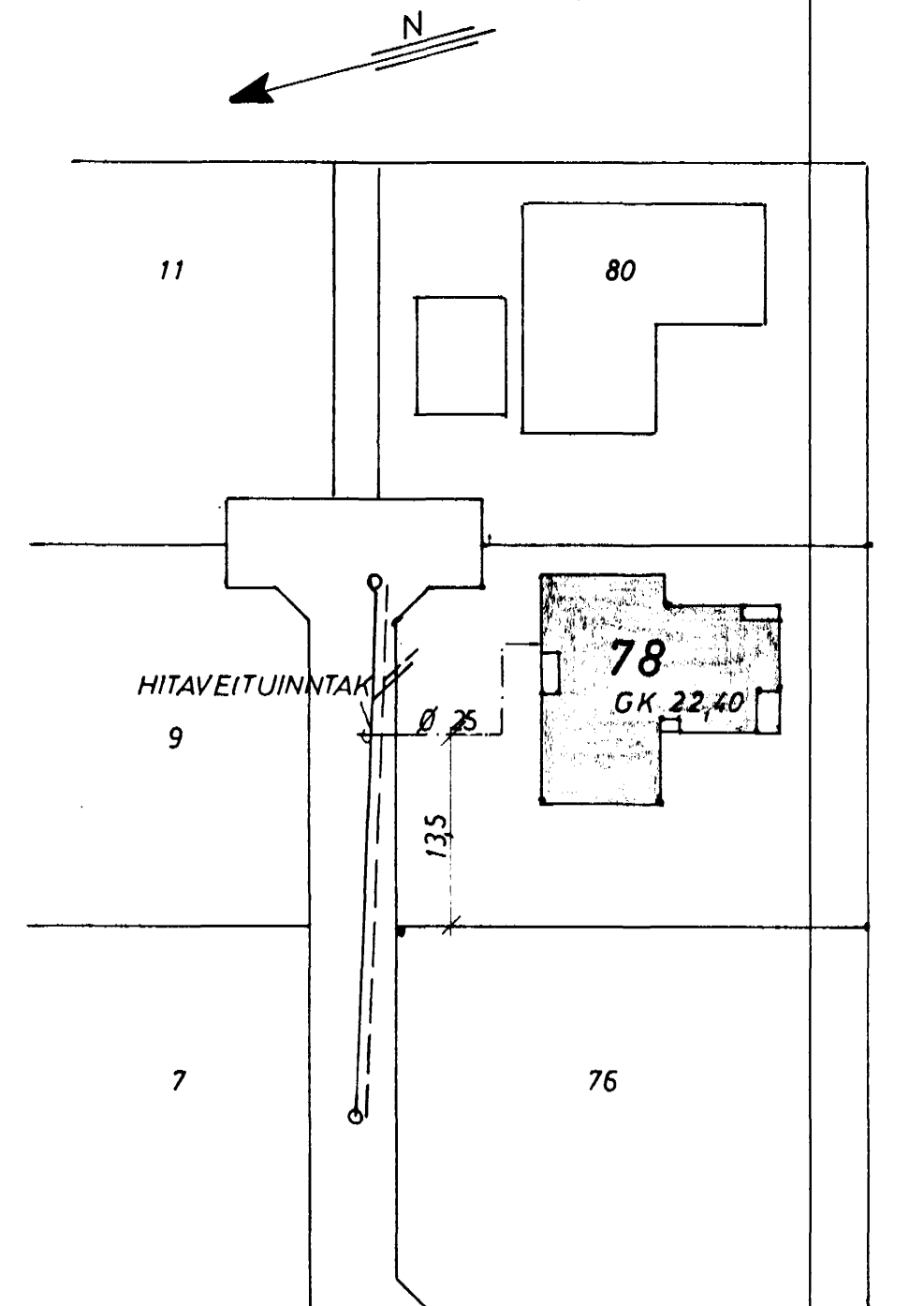
AFSTAÐA 1:500
