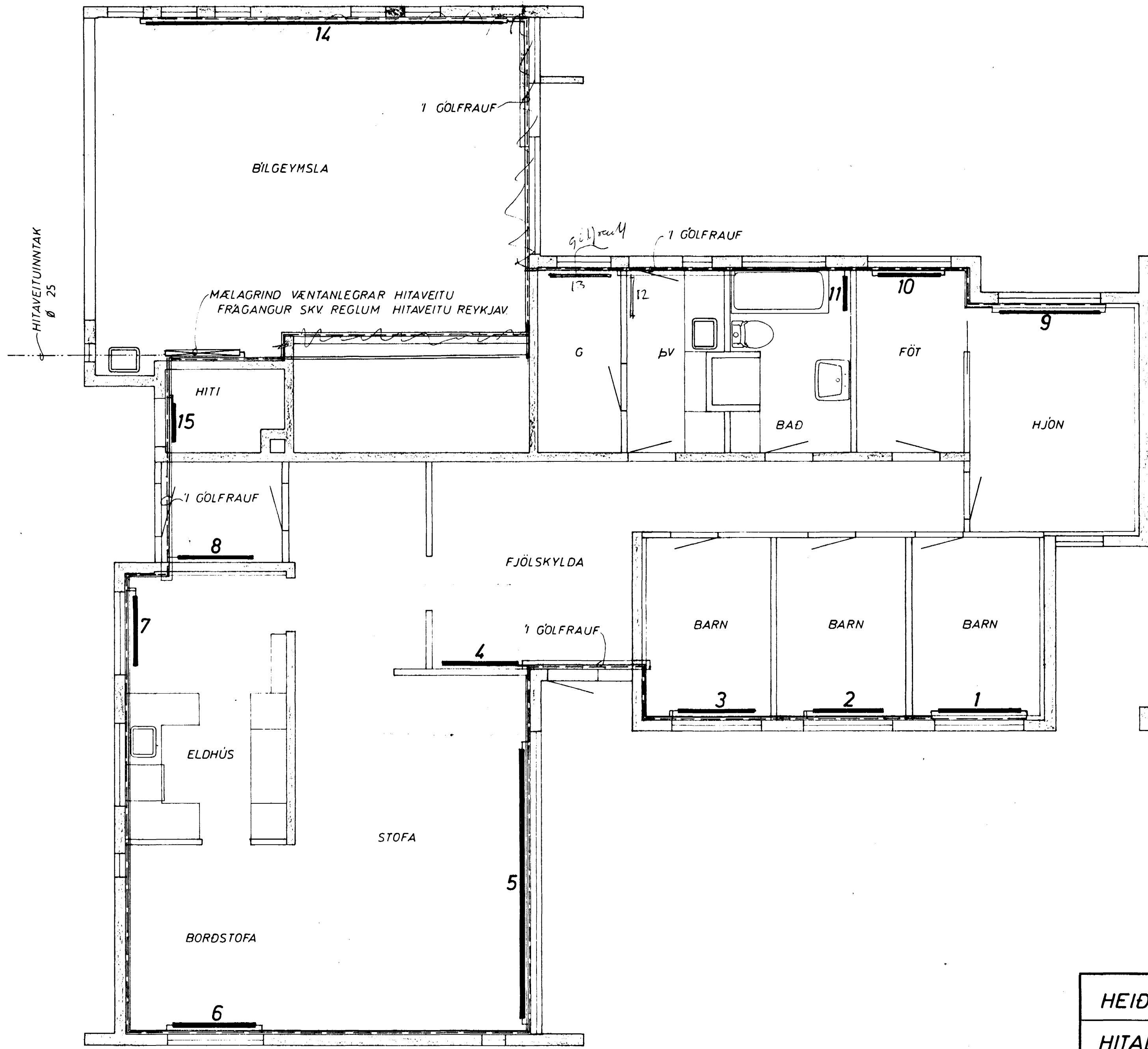
GRUNNMYND 1:50
