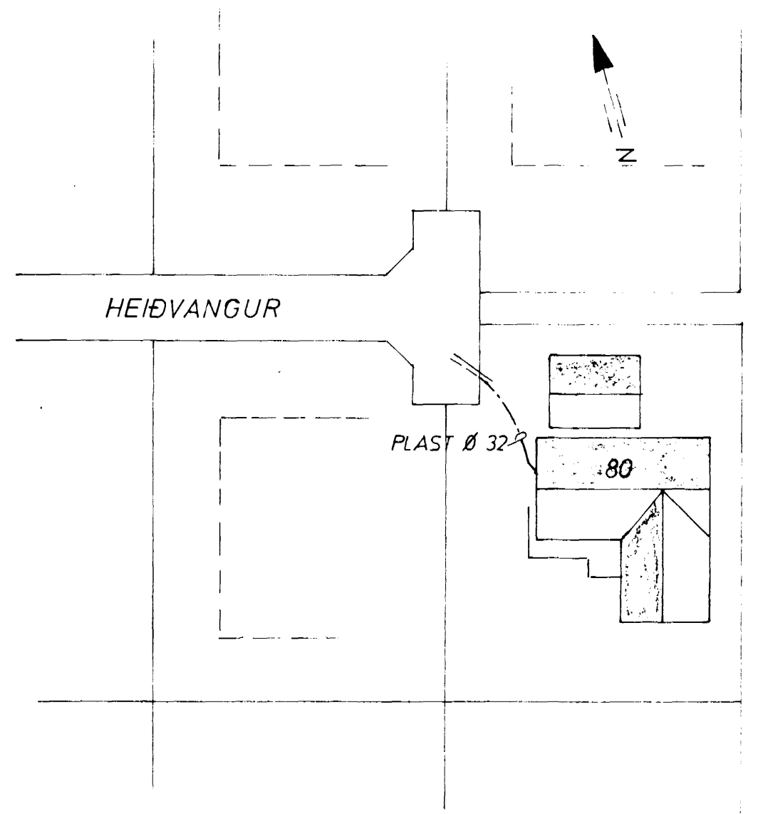
AFSTAÐA 1:500
