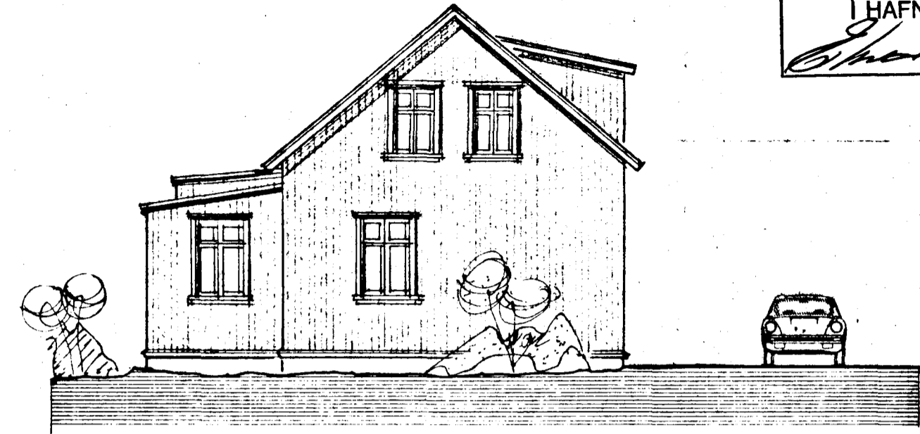
VESTUR 1:100
