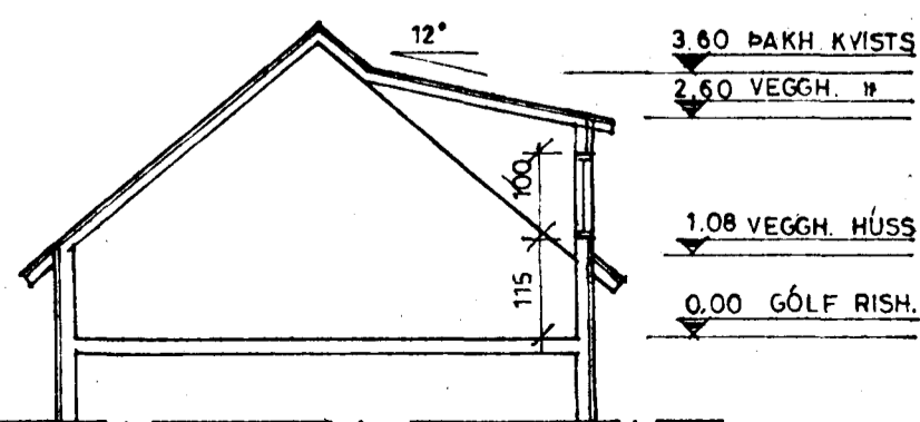
SNÍÐ Í RISHÆÐ 1:100
