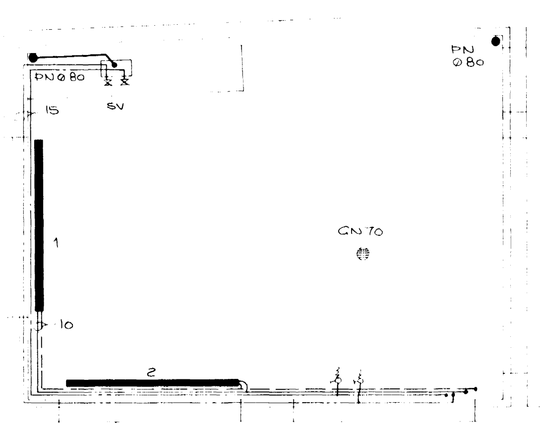
LAGNIR Í BILSKÚR M. 1:50
