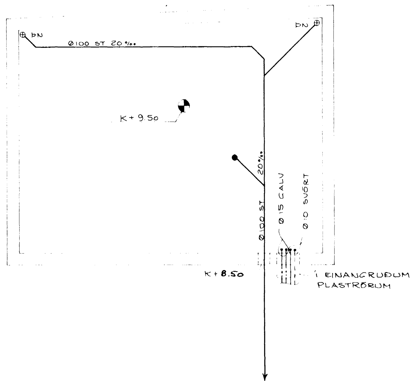
LAGNIR Í GRUNNI M. 1:50
