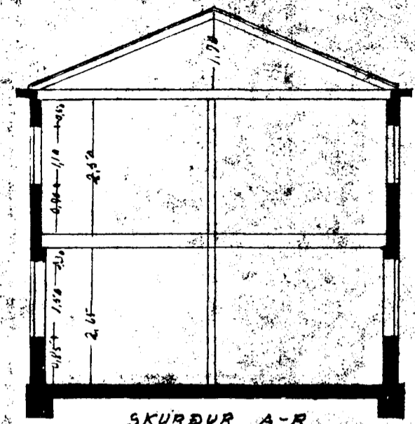
SKURÐUR A-B
