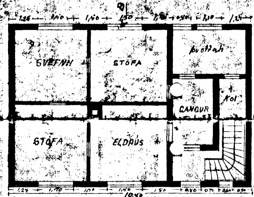
VESTUR
