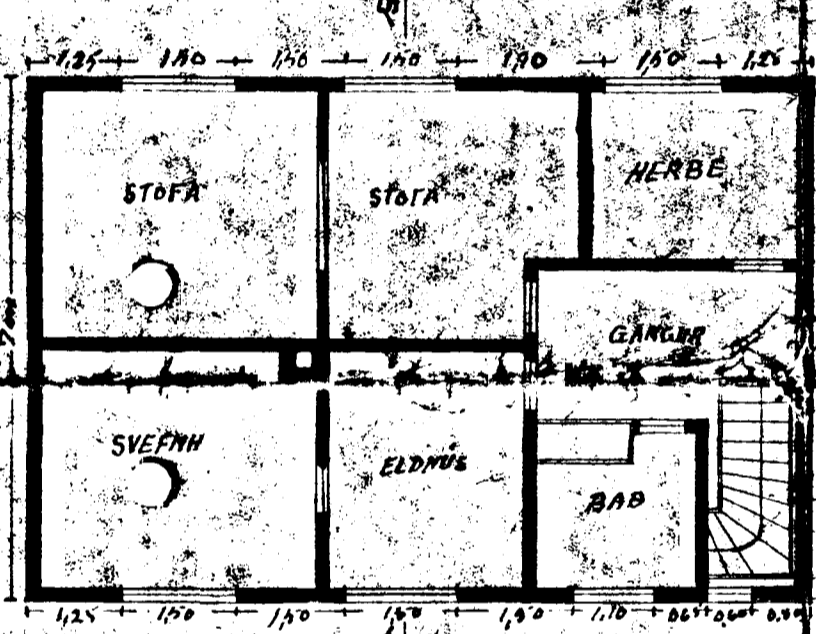
AUSTUR
