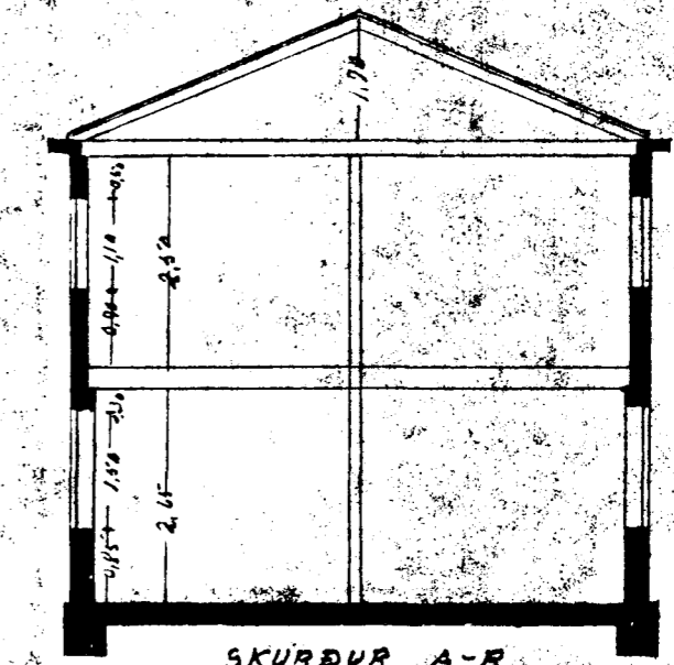
SKURÐUR A-B
