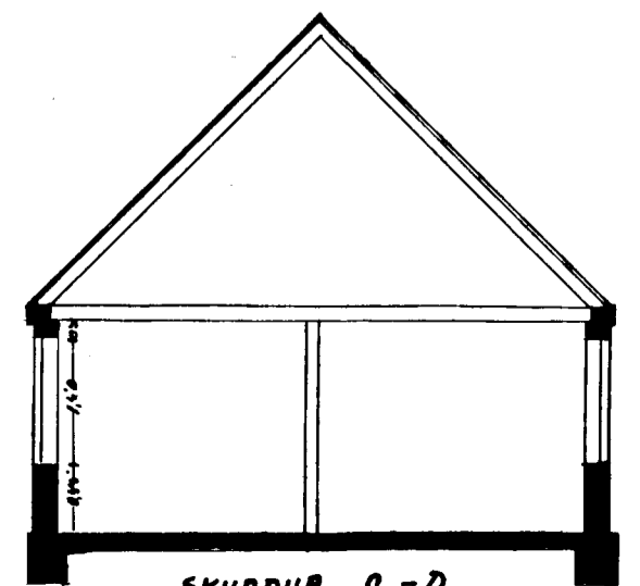
SKURÐUR C-D
