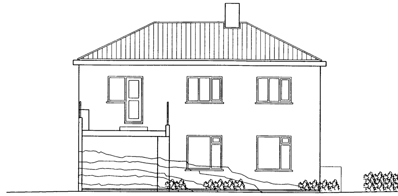
ÚTLIT SUÐVESTUR. MKV. 1:100.
