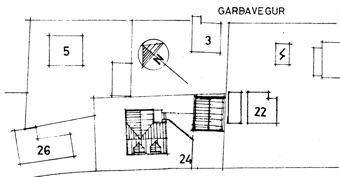
AFSTÖÐUMYND 1:500
