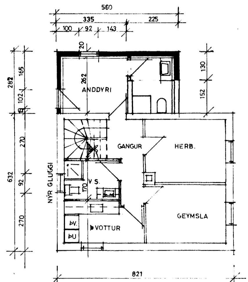
KJALLARI 1:100
