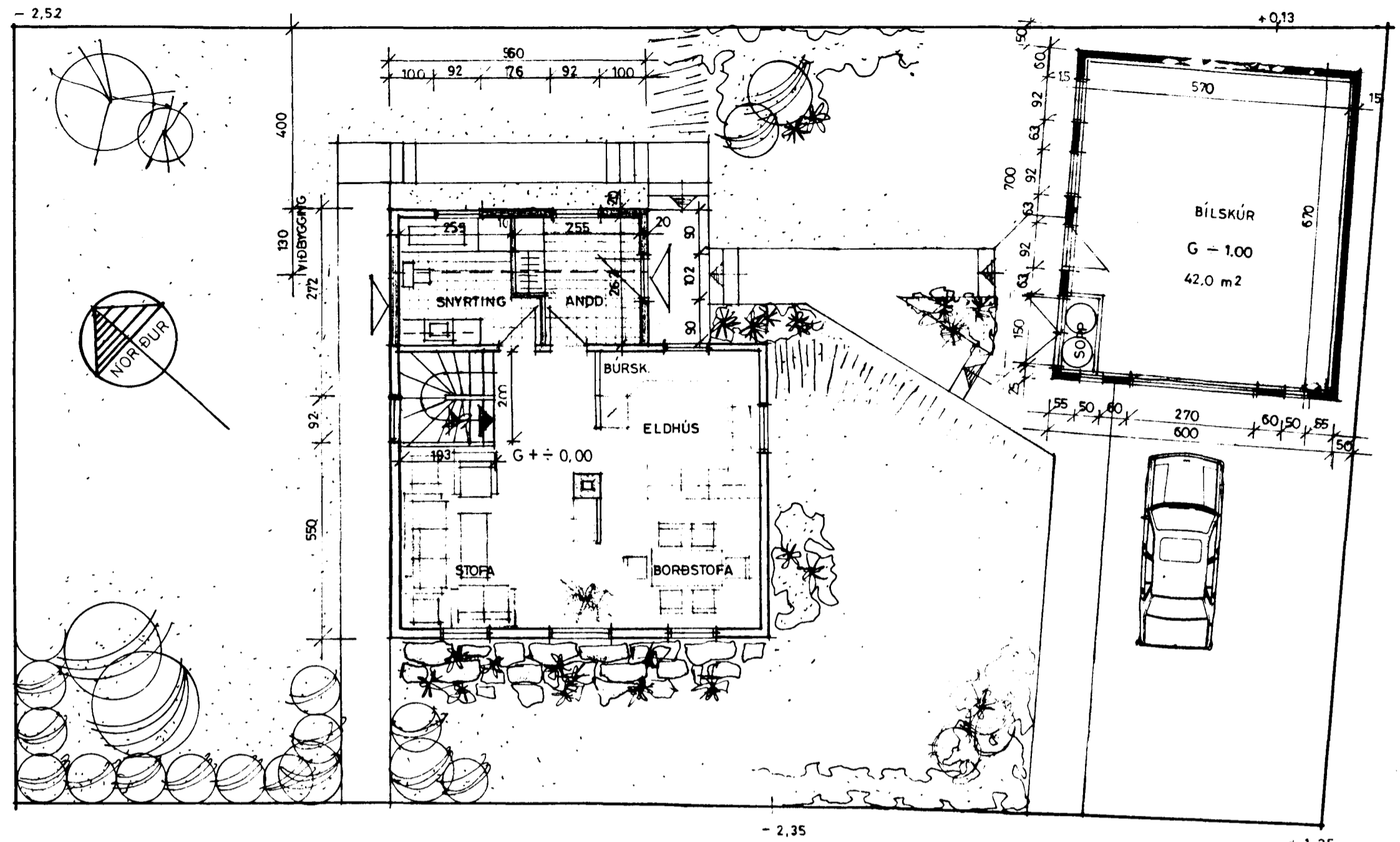
ADALHÆÐ OG LÖÐ 1:100
