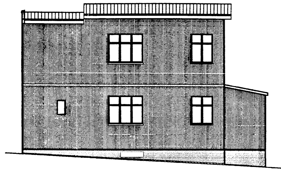
útlit norður
