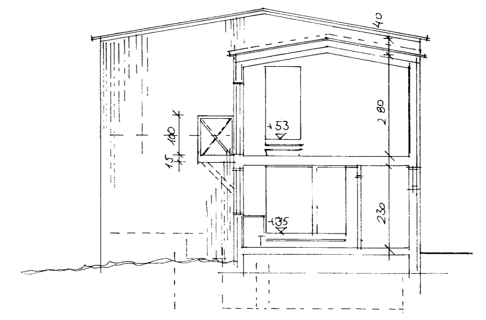
SNEIÐING B-B
