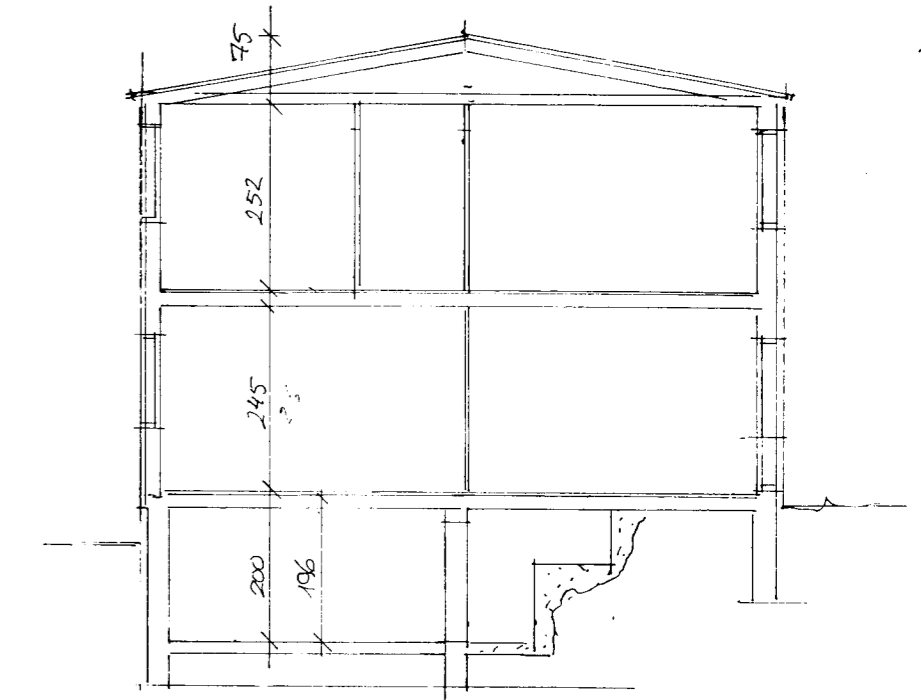
SNEIÐING A-A
