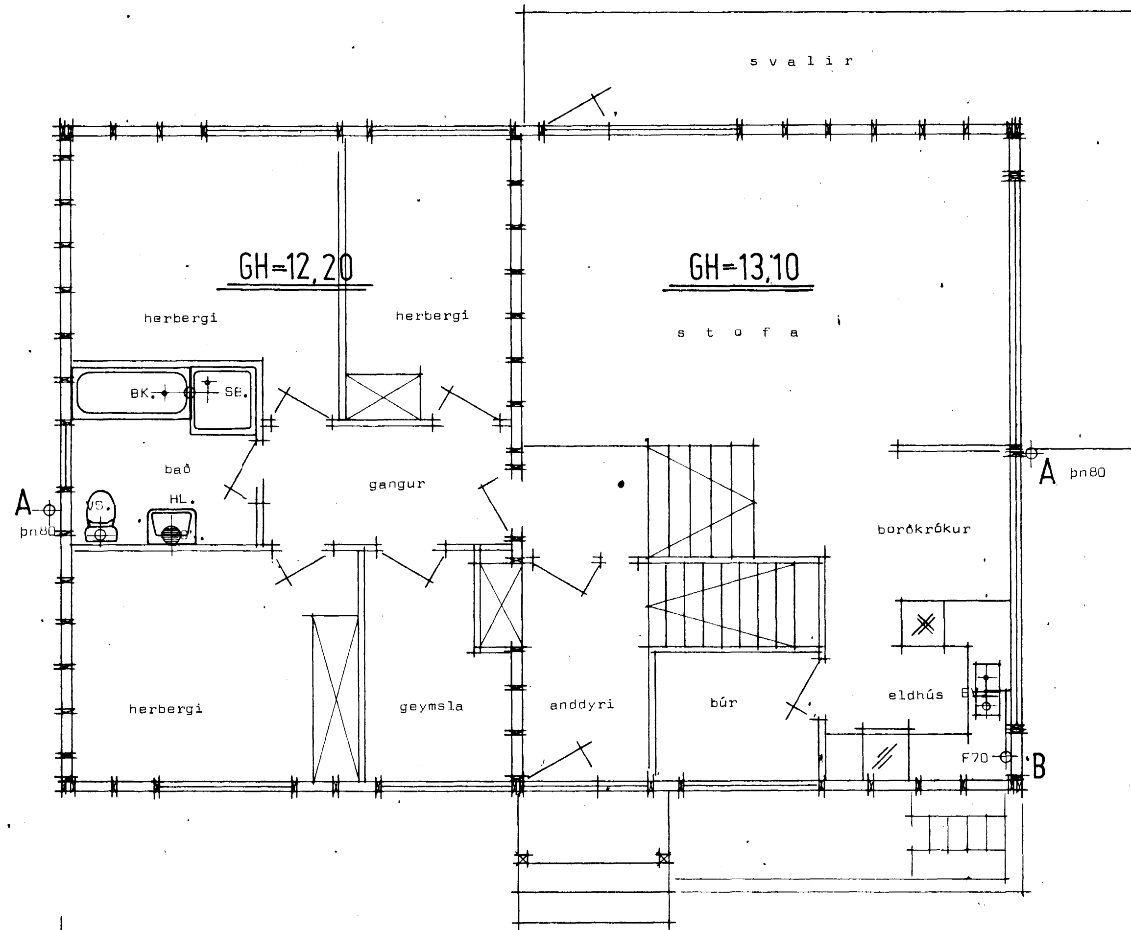
Grunnmynd hæðar Mk 1:50
