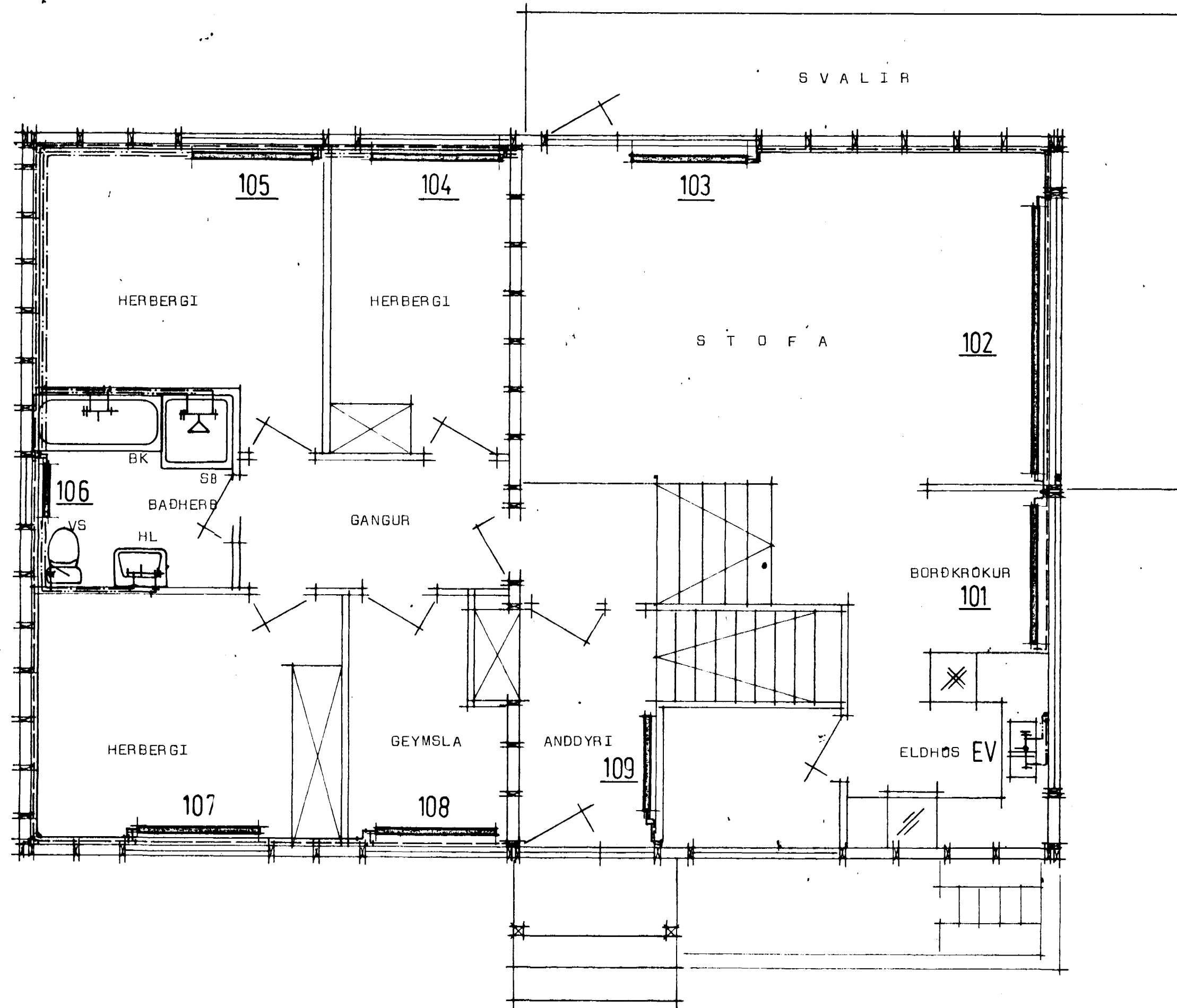
Grunnmynd hæðar Mk 1:50
