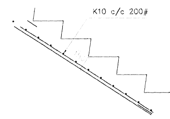
kennisnið stiga 1:20
