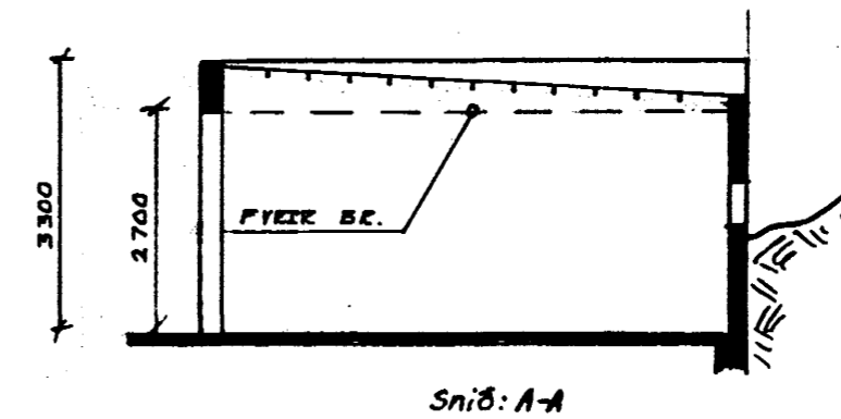
Snið: A-A
