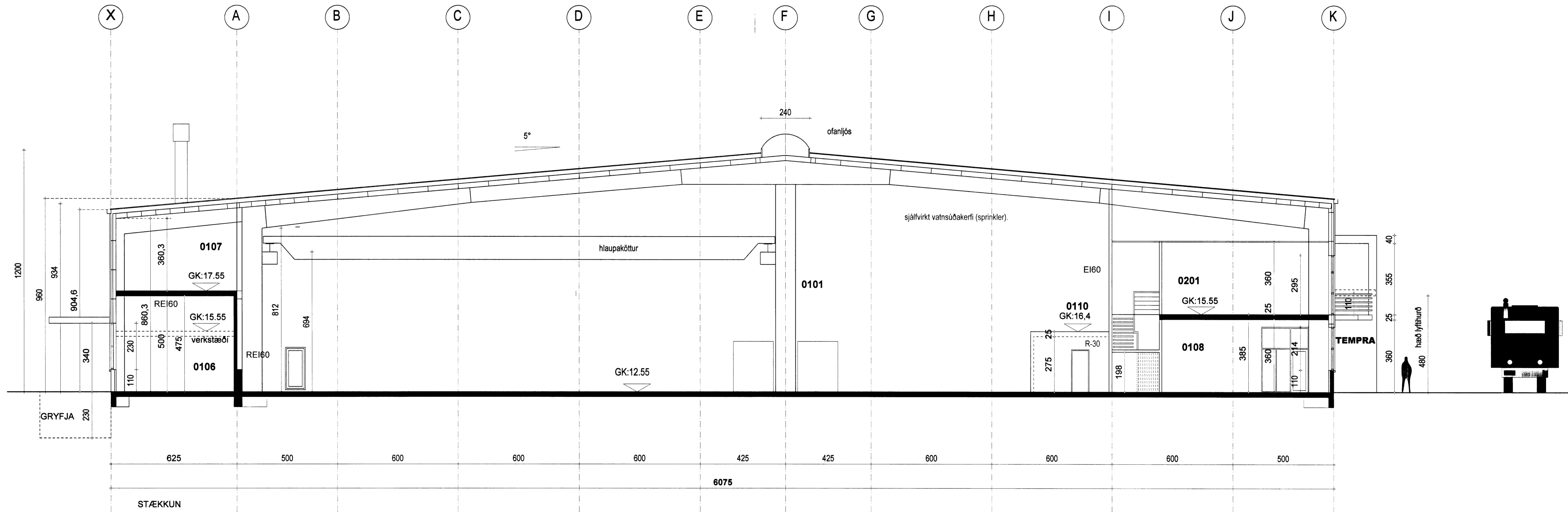
SNEIÐING A-A
