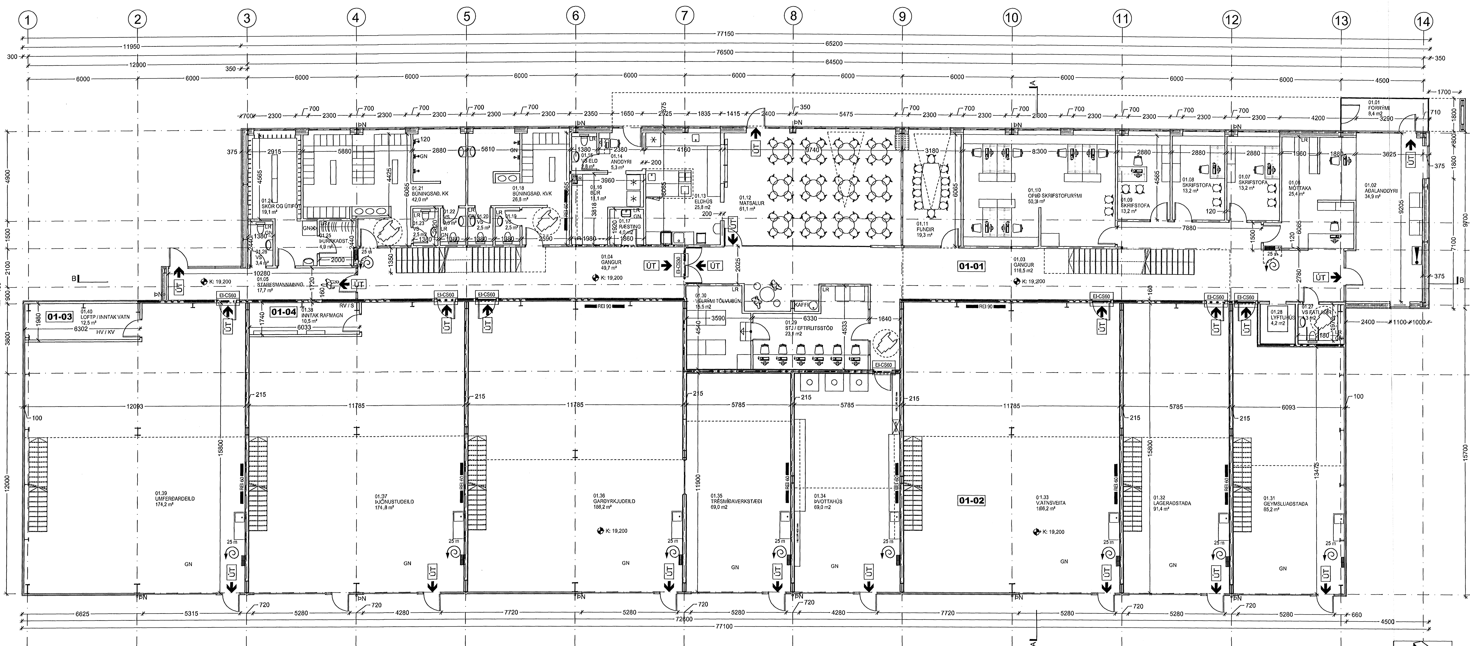
GRUNNMYND 1. HÆÐAR MKV 1:100
