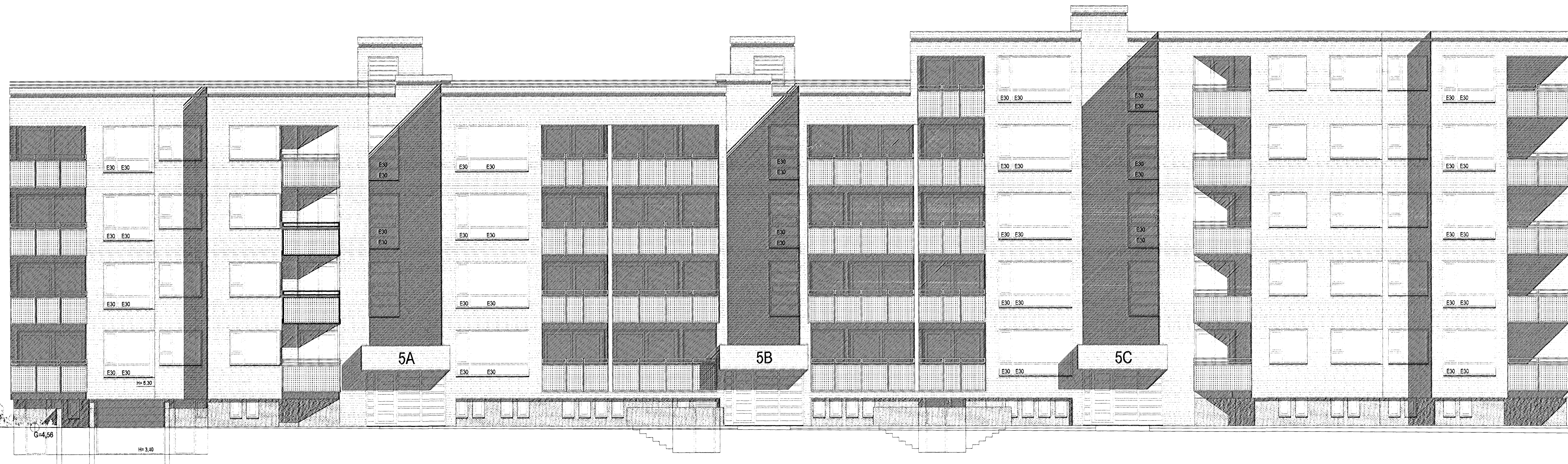
VESTUR. MKV. 1:100.
