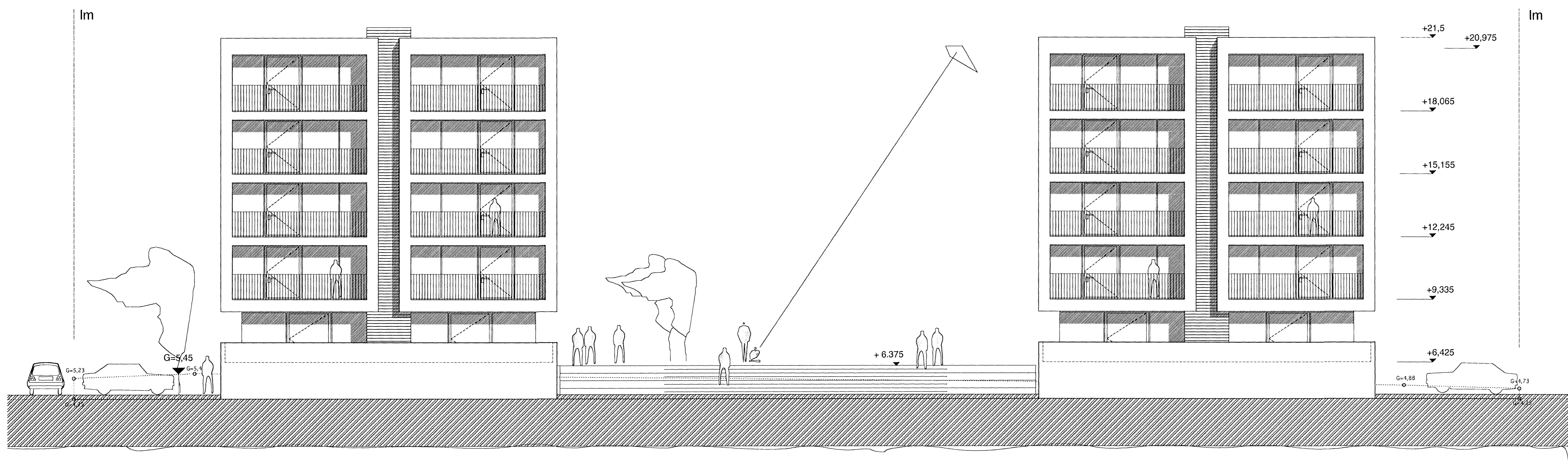
útlit Norðurbakki 9 og 7 - Suður
