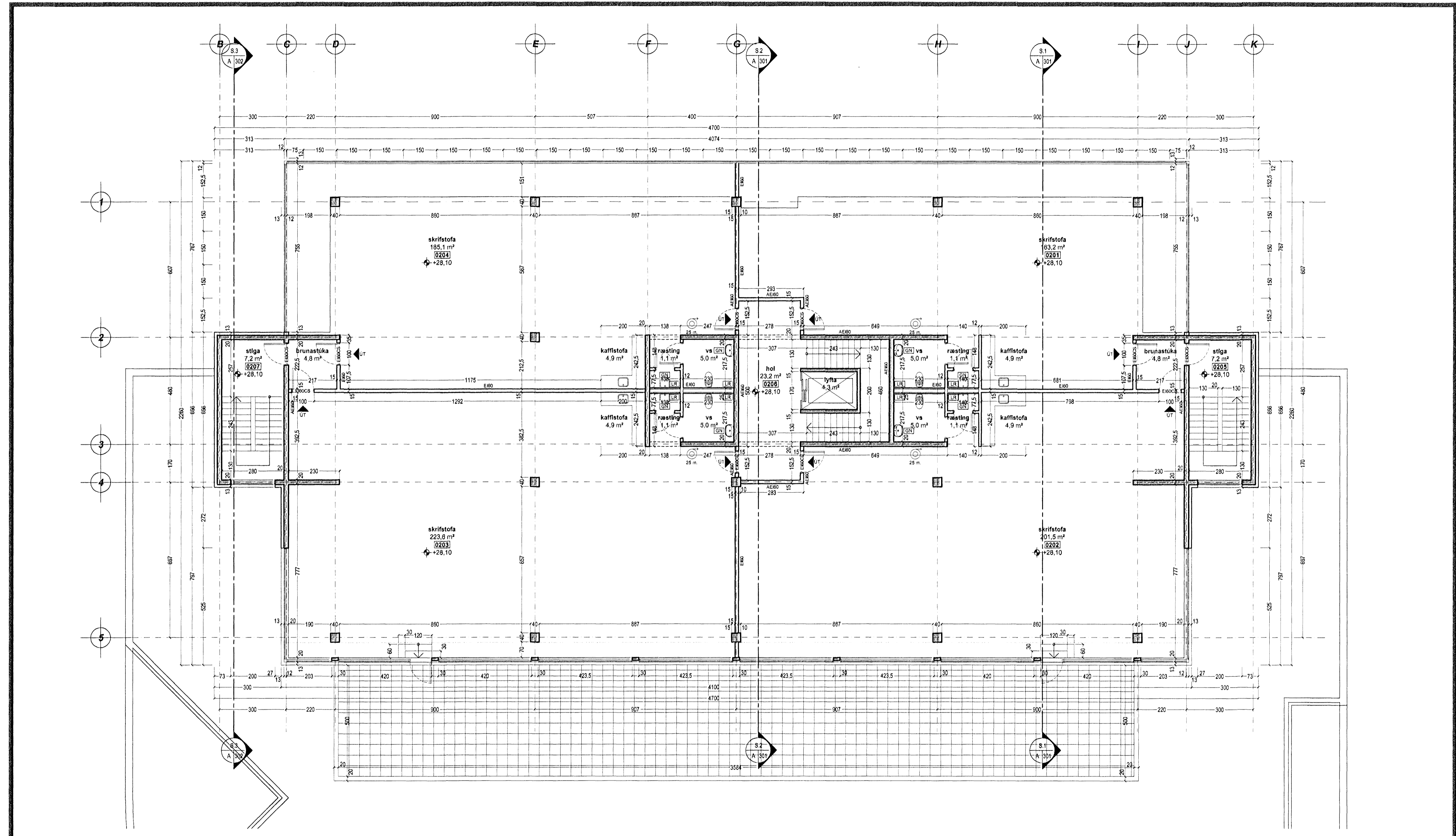
Grunnmynd 2.hæð
