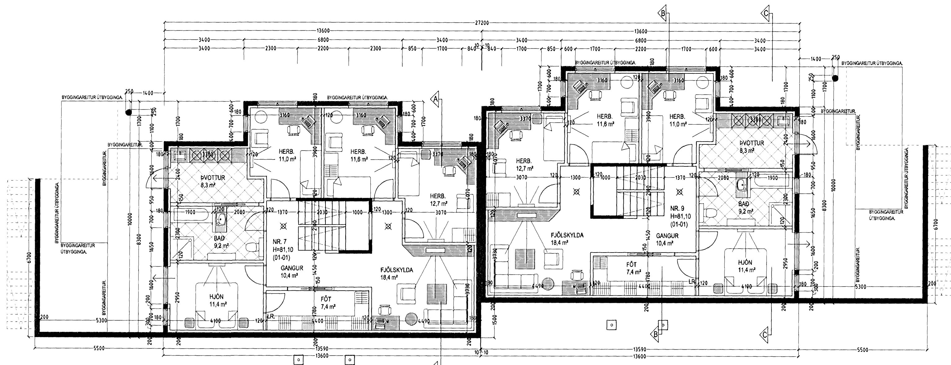
GRUNNMYND 1. HÆÐ MKV. 1:100.
