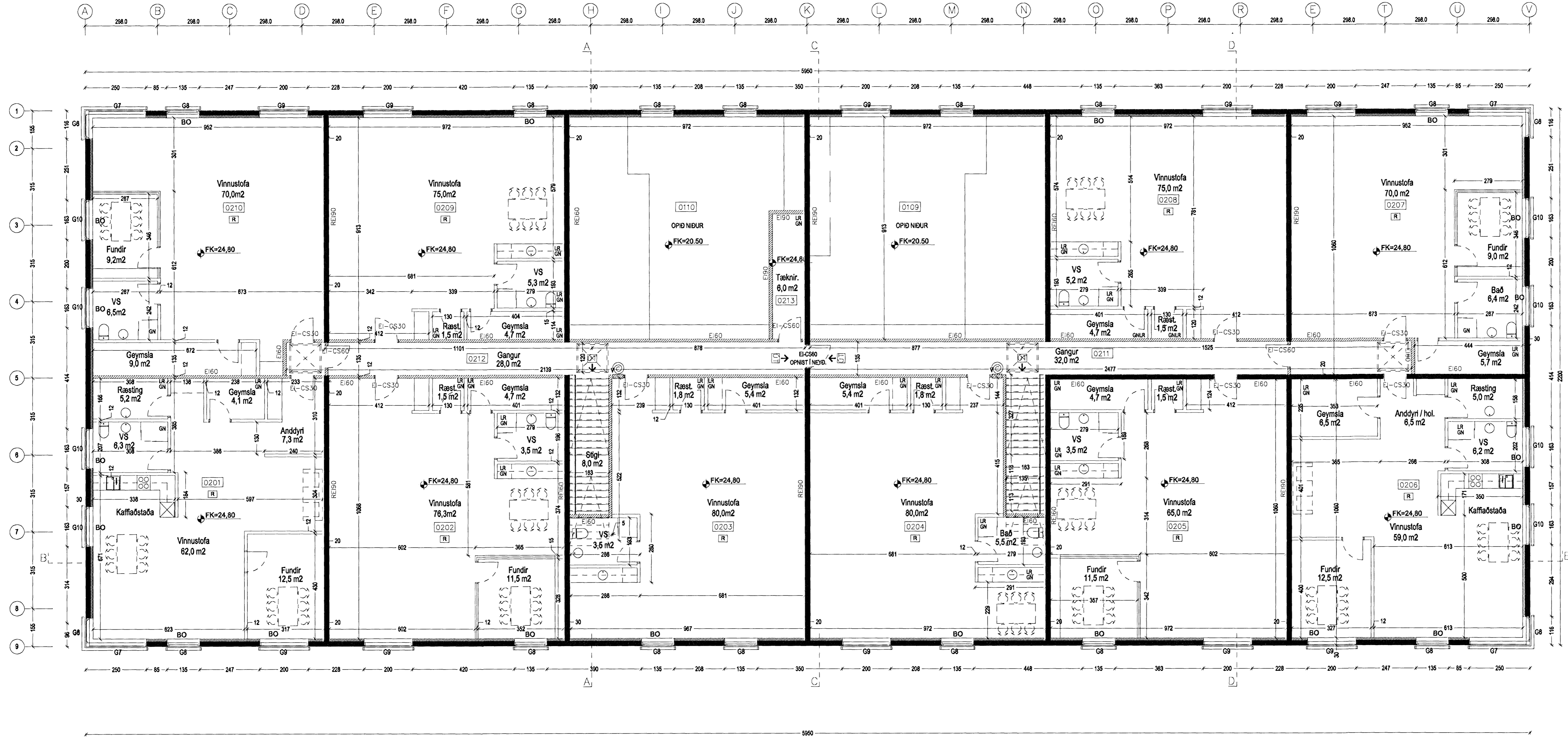
GRUNNMYND 2 HÆÐAR 1:100
