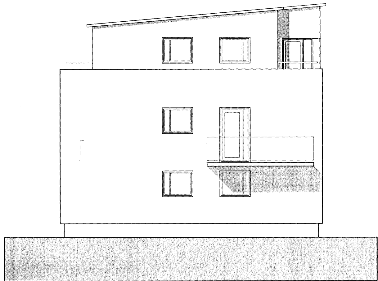
Útlit Norður
