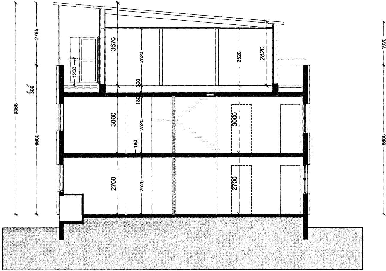
Sníð A-A
