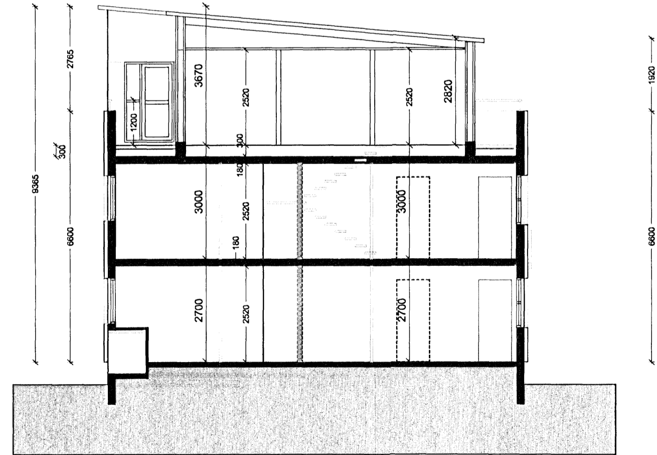
Sníð A-A
