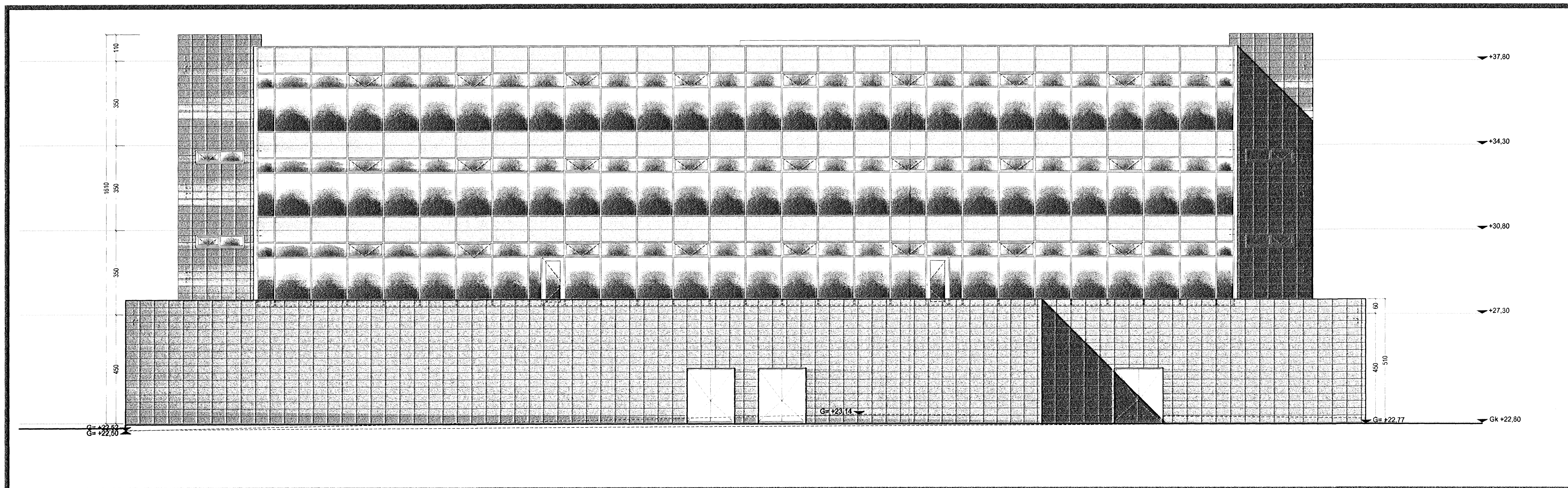
Suður útlit
