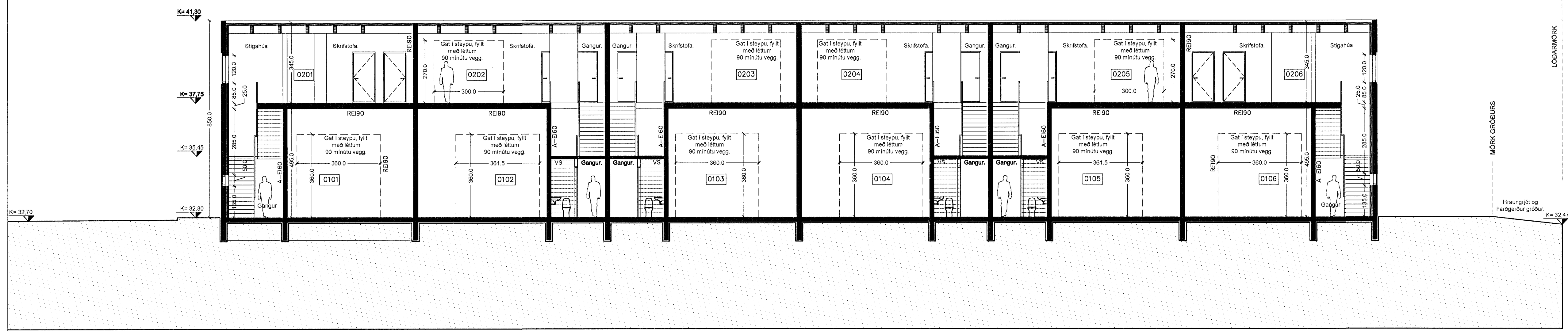
SNÍÐMYND C-C 1:100
