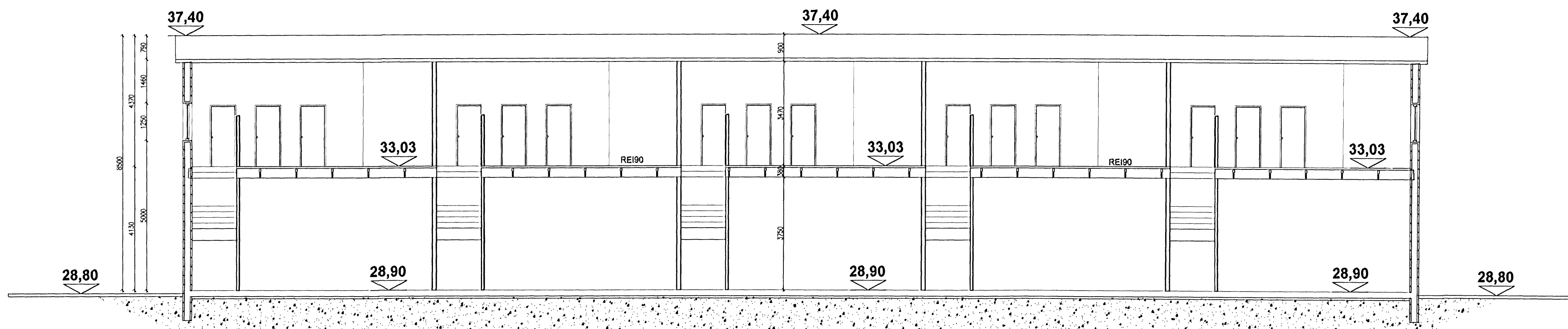
SKURÐUR B-B
