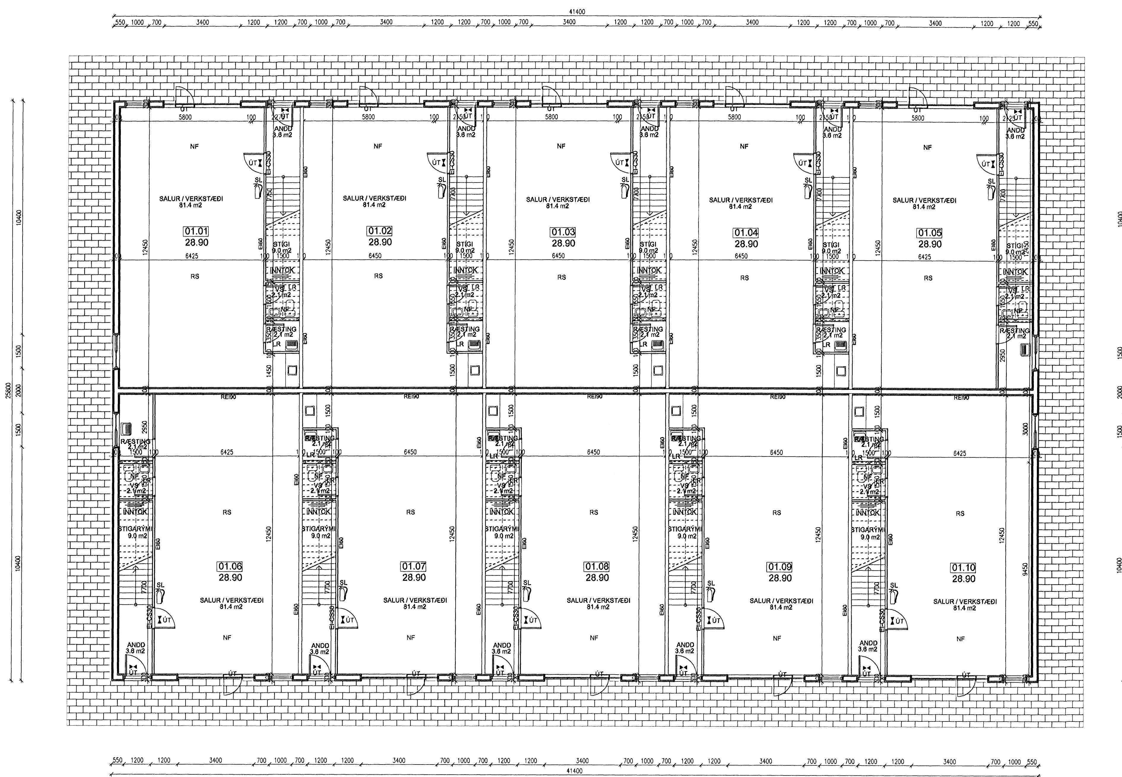
GRUNNMYND 1. HÆÐ
