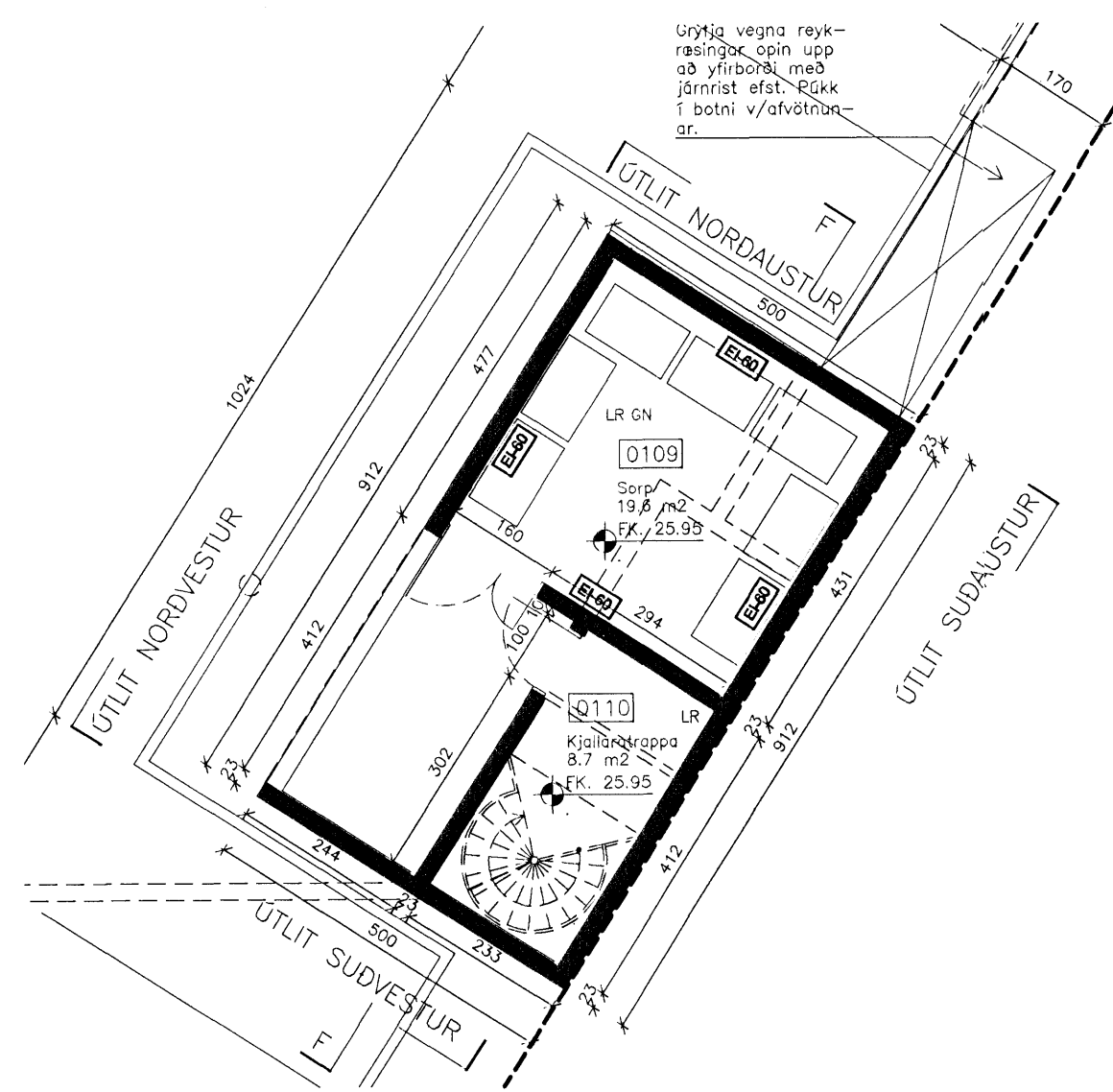
GRUNNMYND SORPGEYMSLU/ FLÓTTASTIGAHÚSS Á LÖÐ
