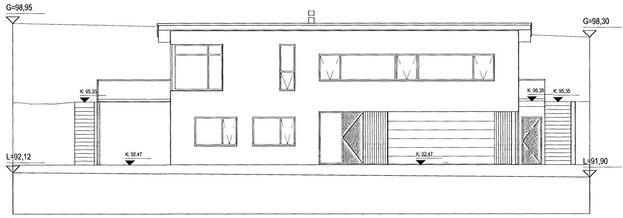
ÚTLIT AUSTUR mkv. 1:100
