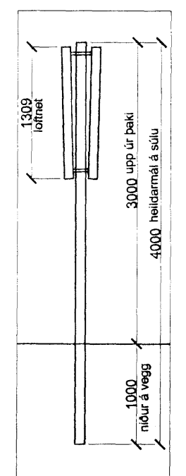
FAR-SÍMA LOFTNET ÁSYND FRÁ HLIÐ
