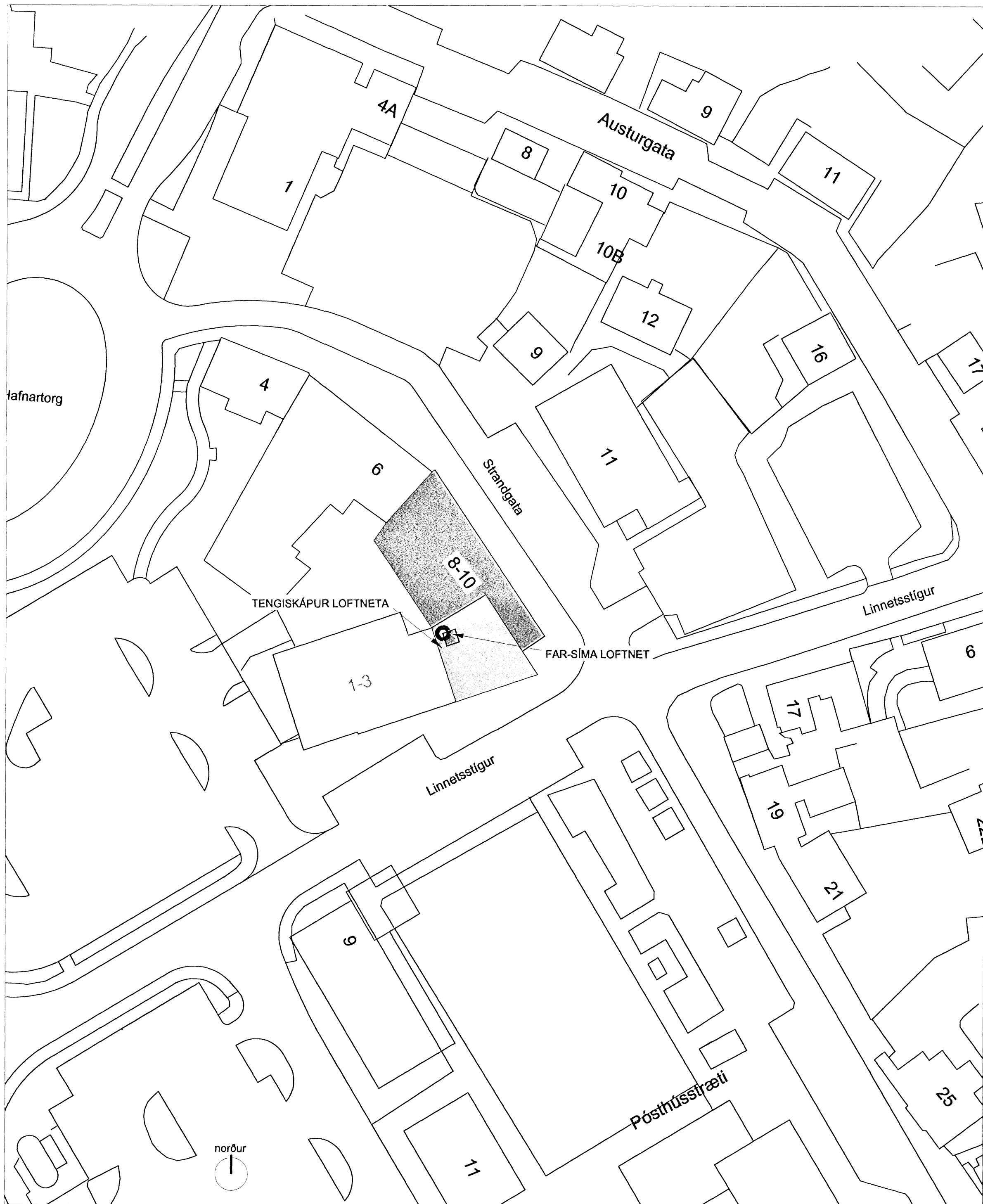
AFSTÖÐUMYND MKV 1:500
