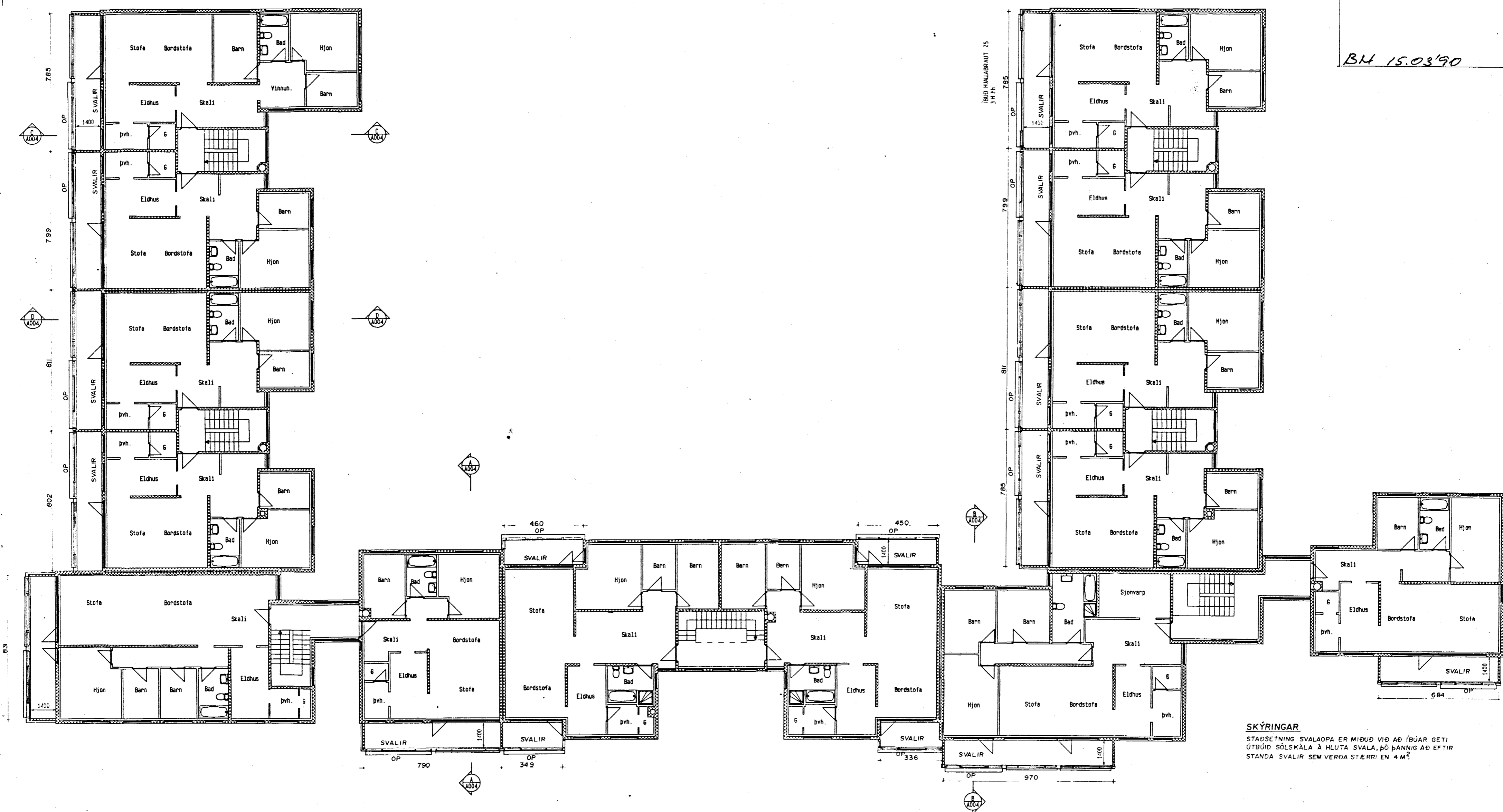
GRUNNMYND SVALA 3. HÆÐ 1/100
