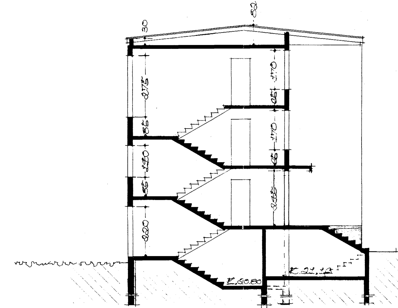
SNIÐUR B-B
