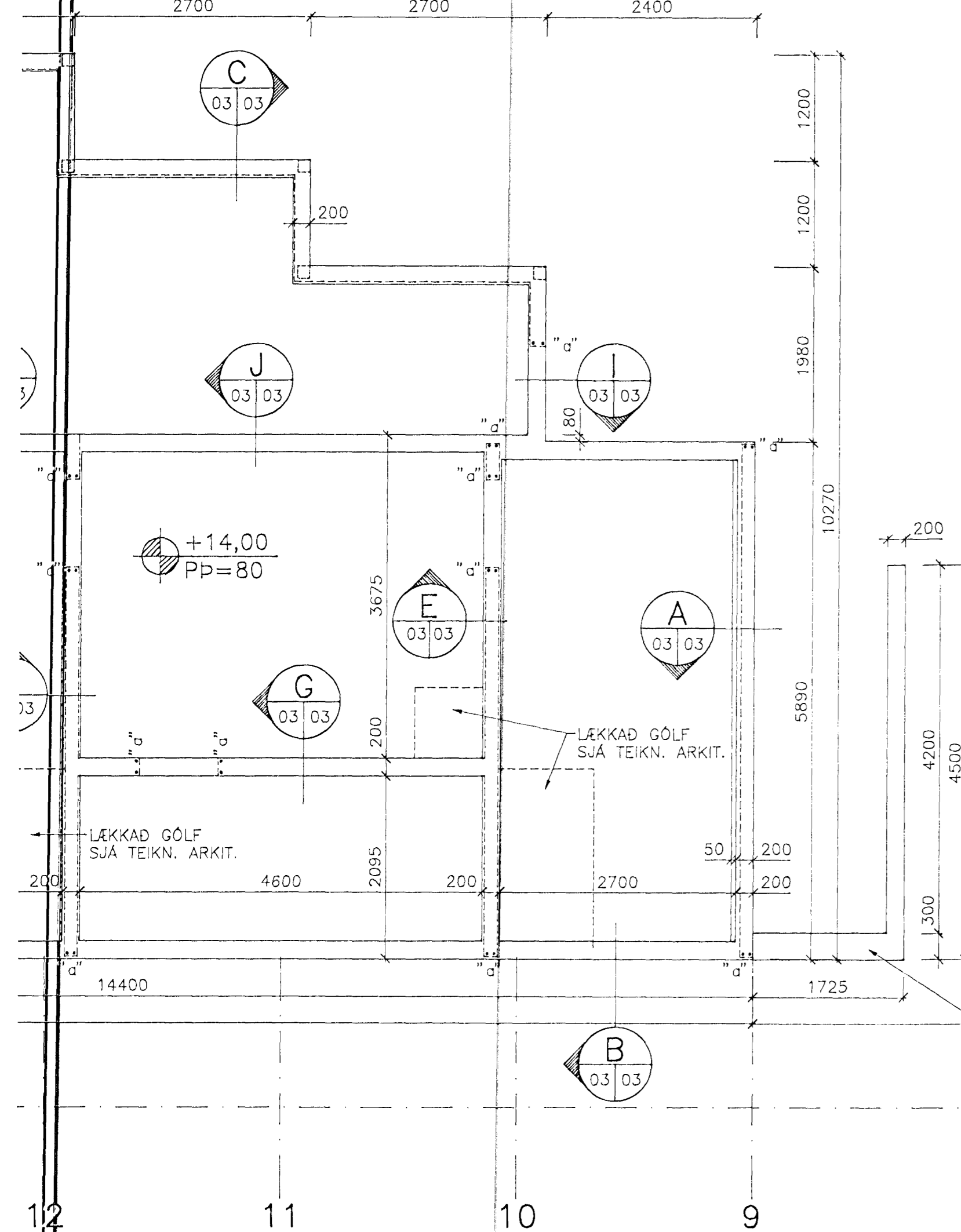
GRUNNMYND, SUDUR HLUTI 1:50
