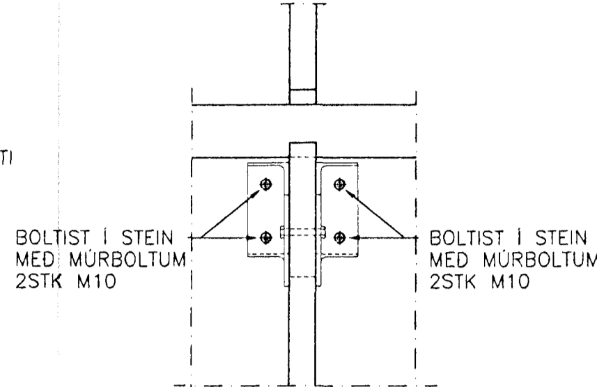
SNID XVIIIa-XVIIIa 1:10
