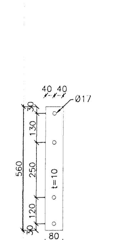
FESTING F10 1:10
