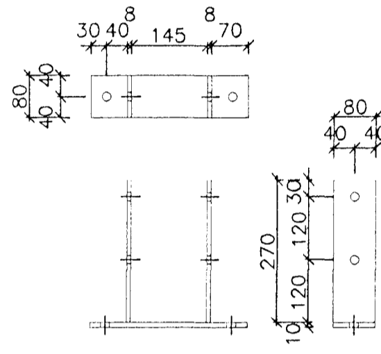
FESTING F11 1:10
