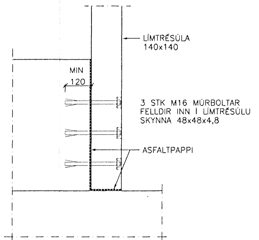
SNID XXVIIa-XXVIIa 1:10
