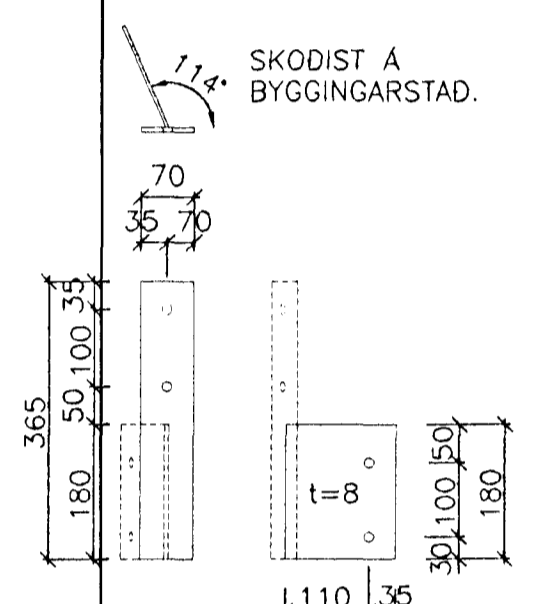
FESTING F12 1:10
