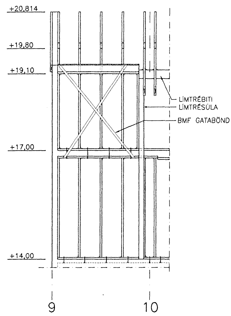
H SNID M. 1:50
