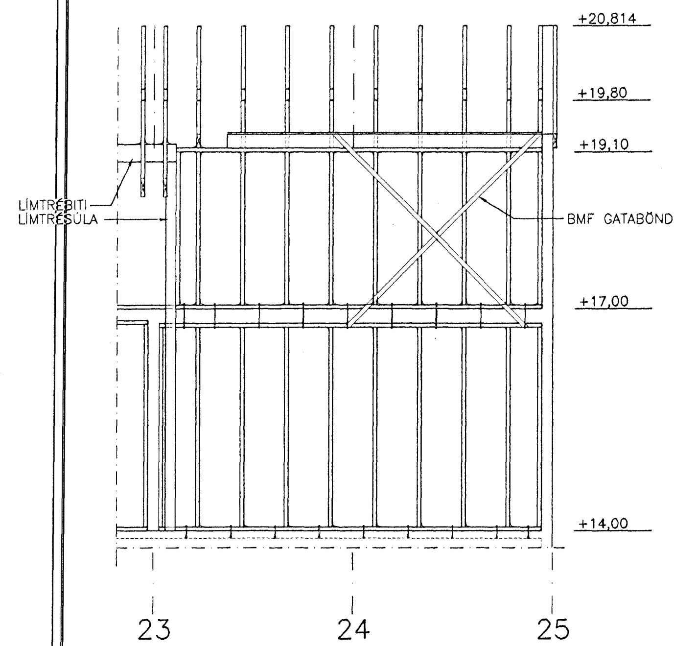
G SNID M. 1:50
