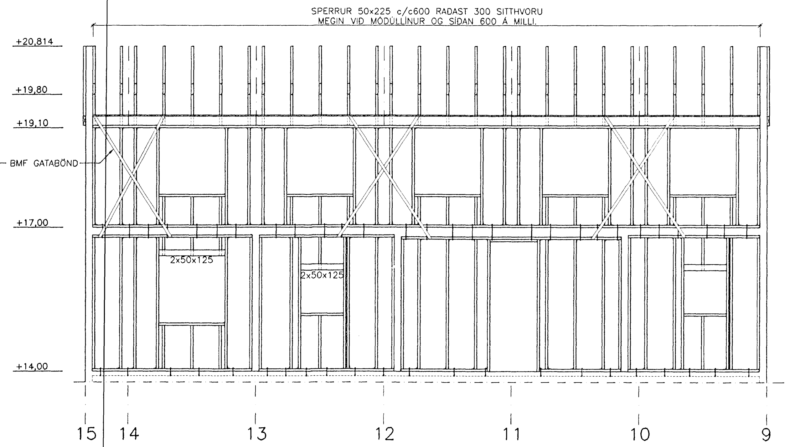
F SNID M. 1:50
