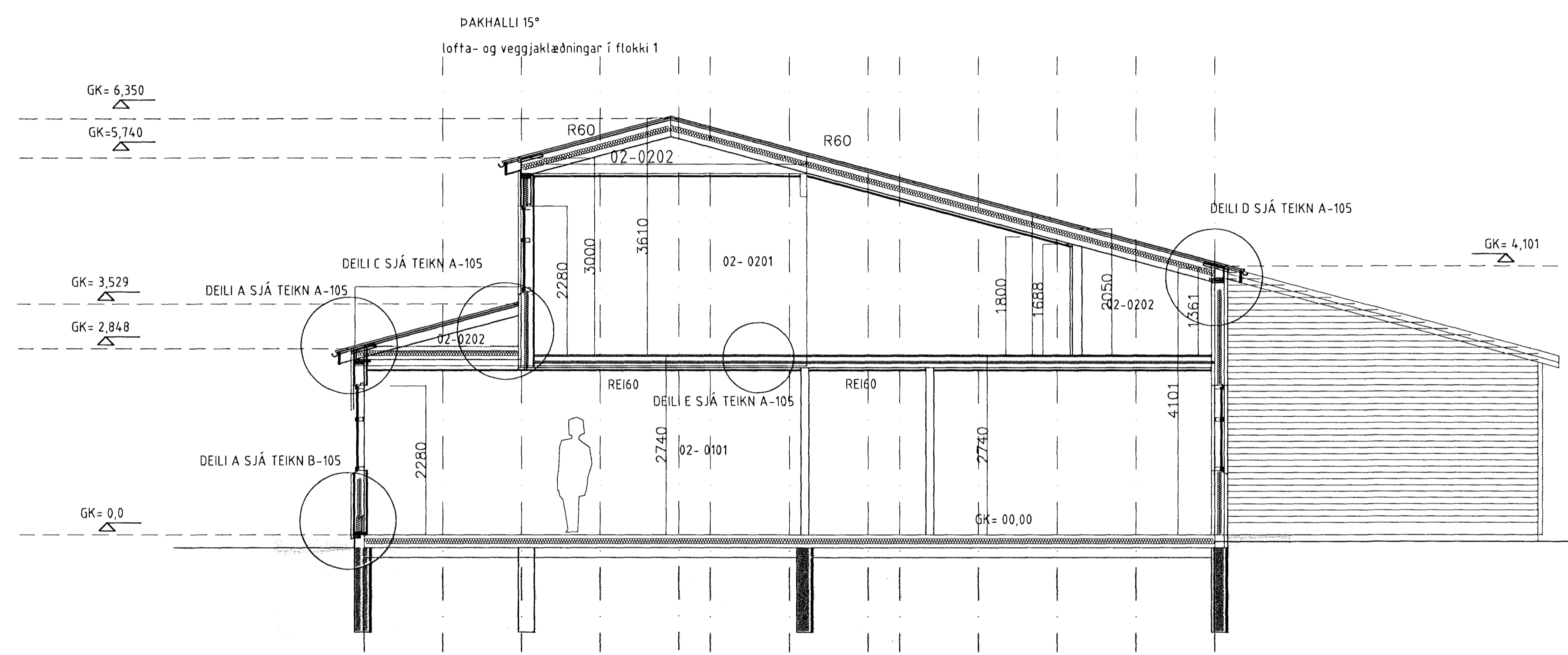
SNEIÐMYND B-B
