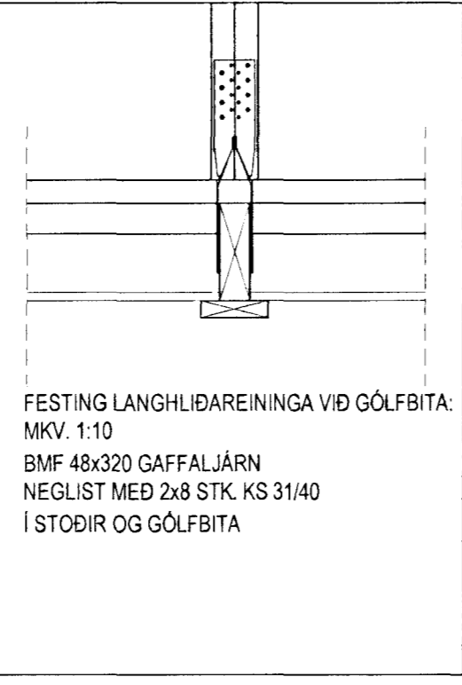
F15 FESTING F15 MKV. 1:10
