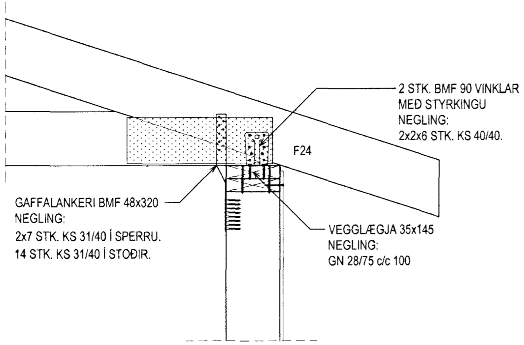
F24 FESTING F24 MKV. 1:10
