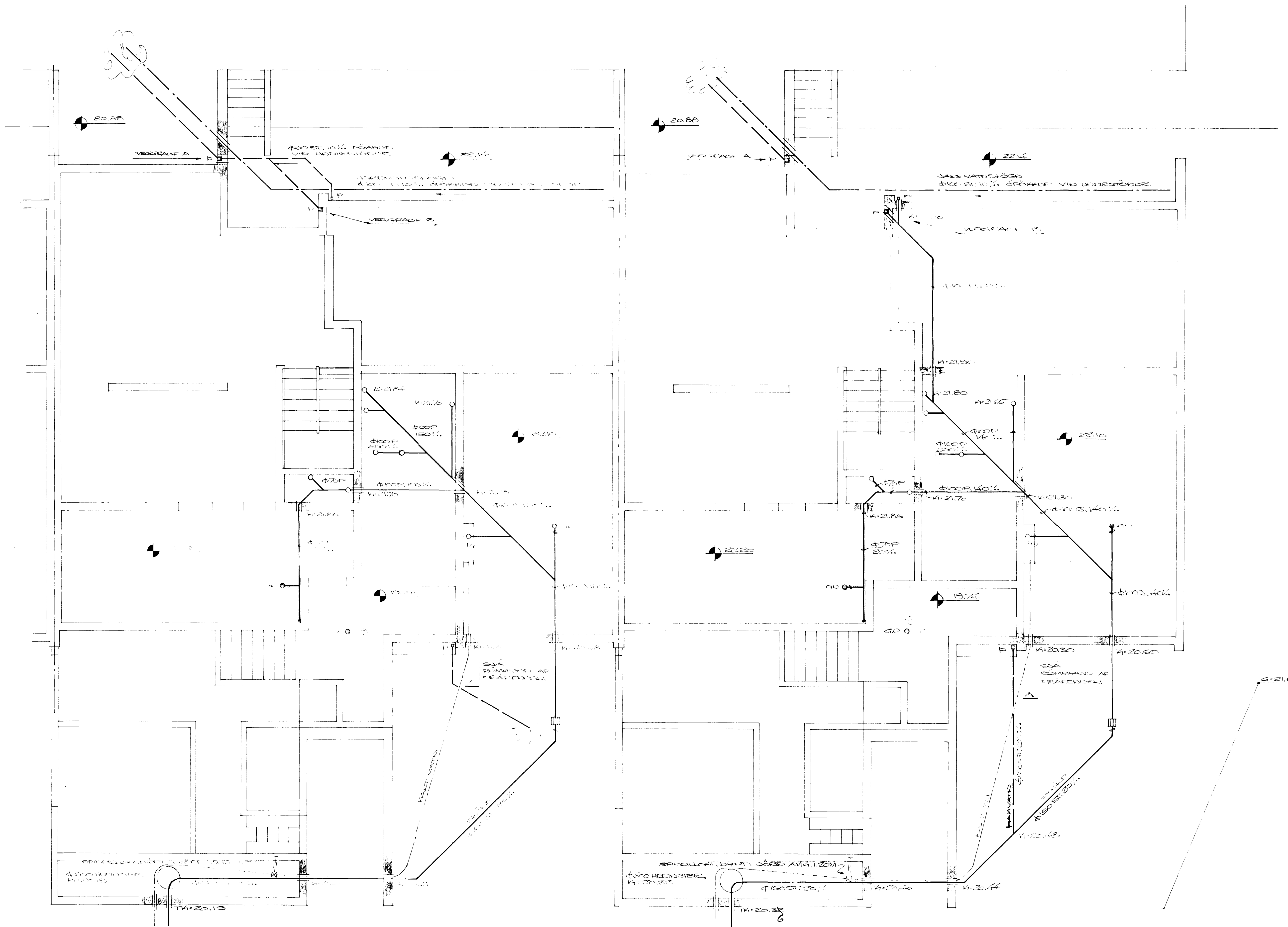
GRUNDRISSD. M=1:800
