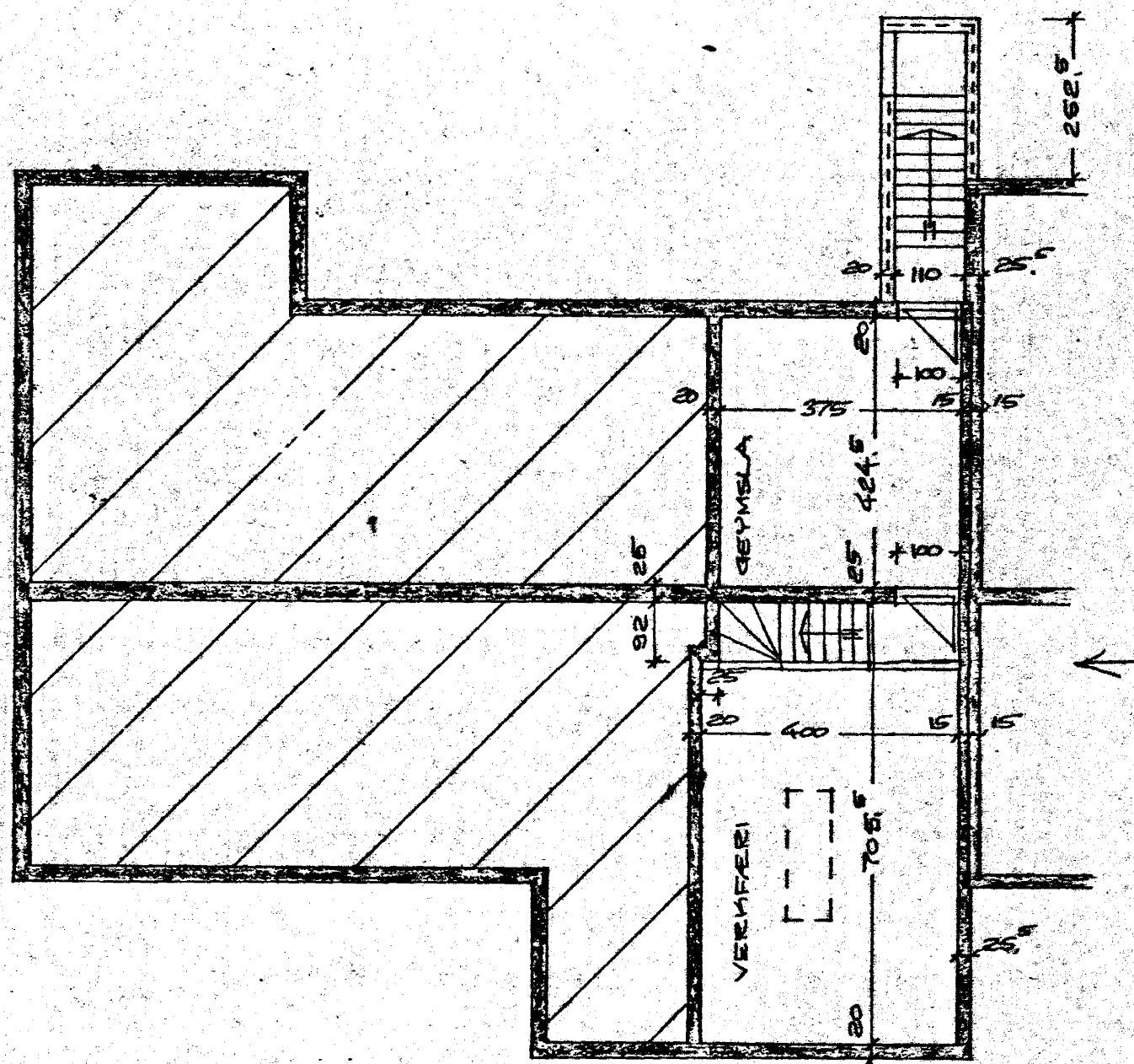
GRUNNMYND KJALLARA
