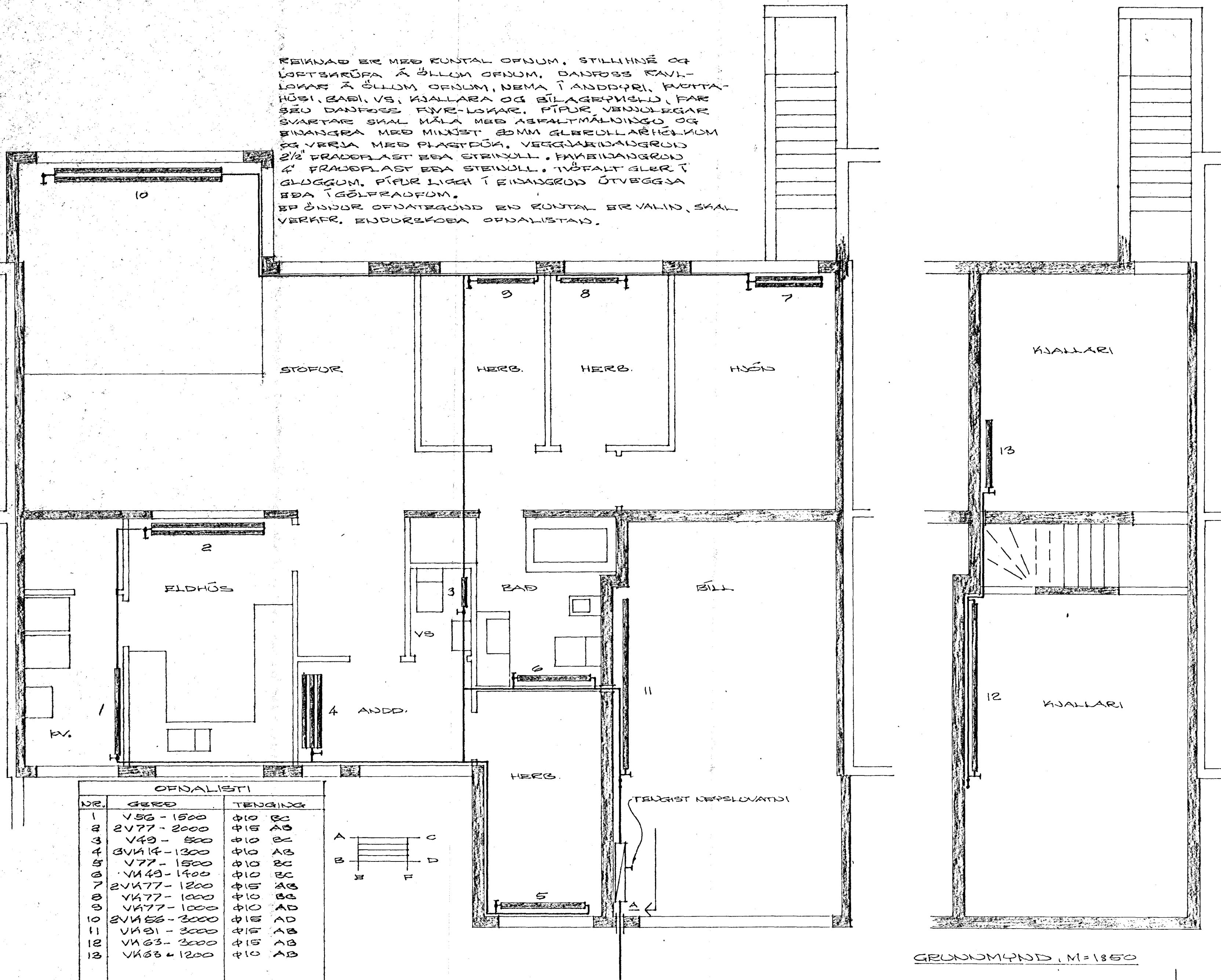
GRUNNMYND, M=1:50
