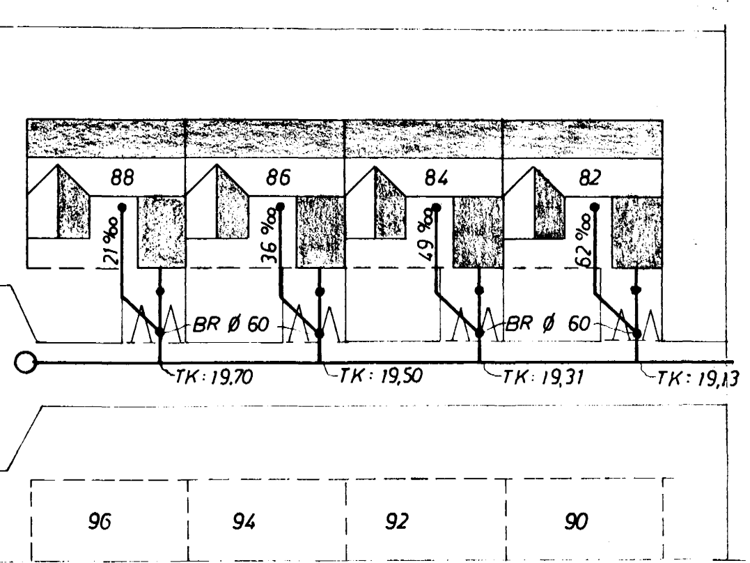
AFSTADA 1:500
