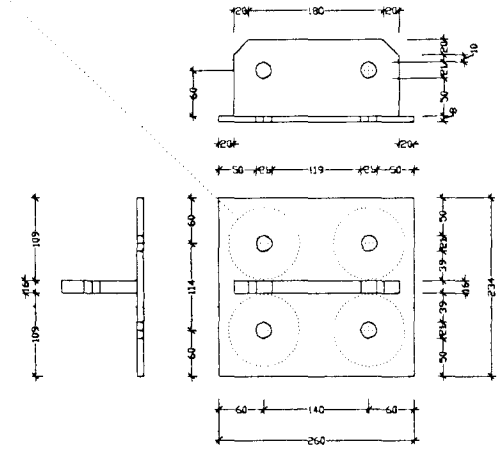
Stálfesting VSp.1. Vindstífung í þaki. 4 samsetningar. 4 stk.
