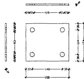
Stálfesting VSp.1. Vindstífung í þaki. 4 samsetningar, laskar. 4 stk.
