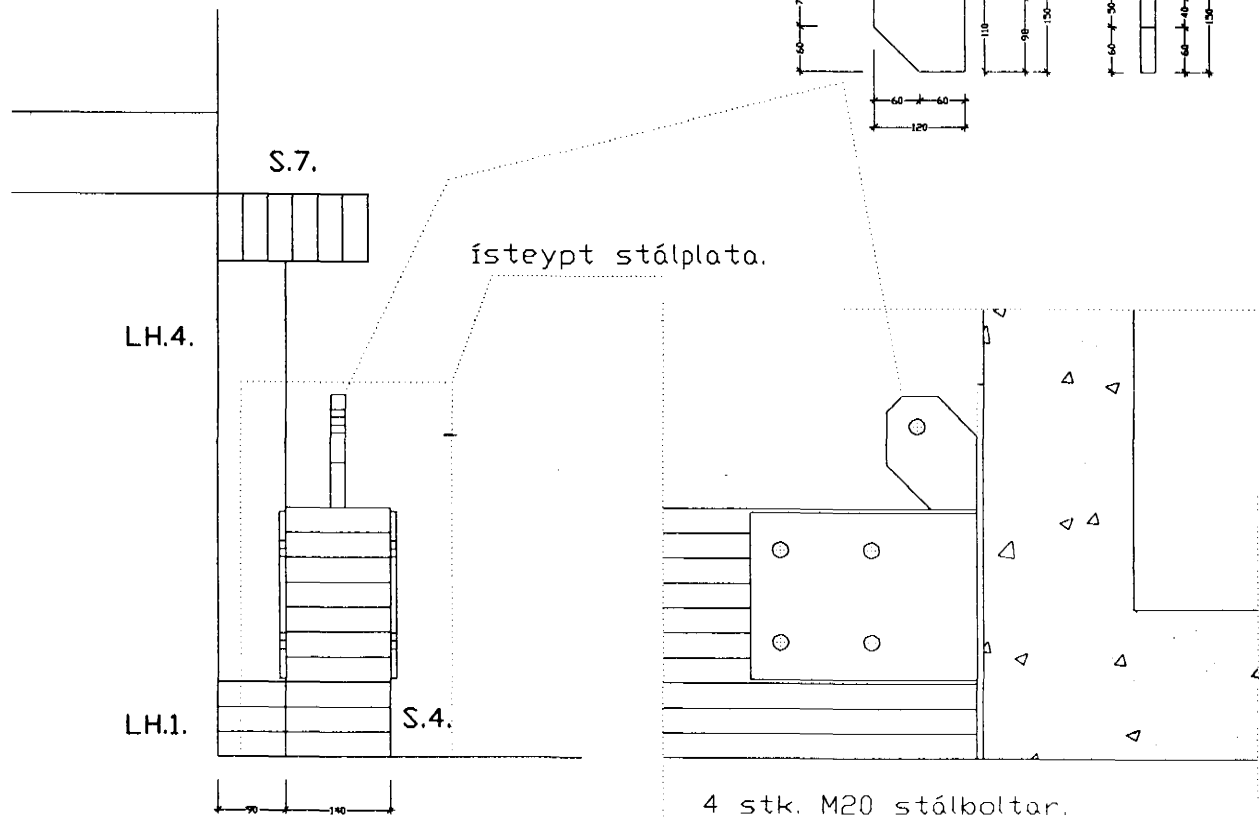
STÁLFESTING AF.1. HORNSOLA. Ein súla. Stálfesting soðin á staðnum á ísteypa stálplötu.
