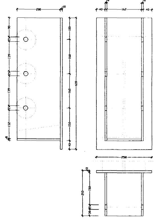
STÁLFESTING FF. 3 stk. 3 samsetningar. Stálfesting soðin á staðnum á IPE 500 þakbita.
