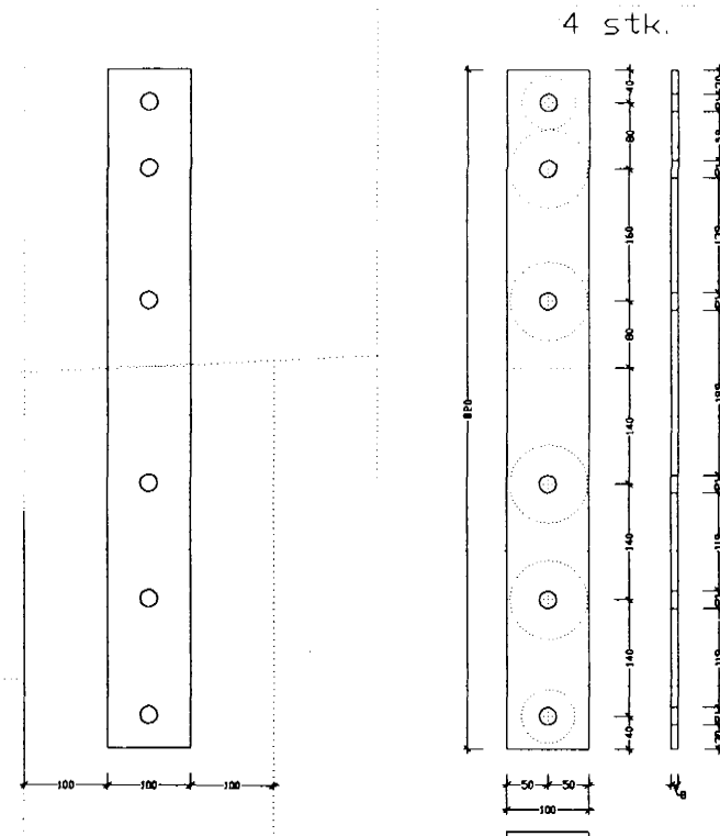
Stálfesting EF. 2 samsetningar. Sjá einnig VSV.3.
