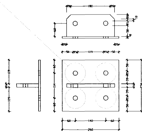
Stálfesting VSp.1. Vindstífung í Paki. 4 samsetningar. 4 stk.
