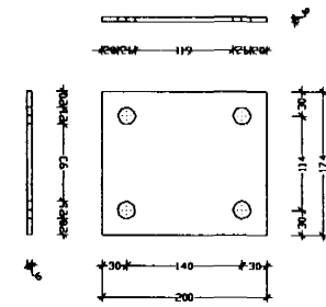
Stálfesting VSp.1. Vindstífung í Paki. 4 samsetningar, laskar. 4 stk.
