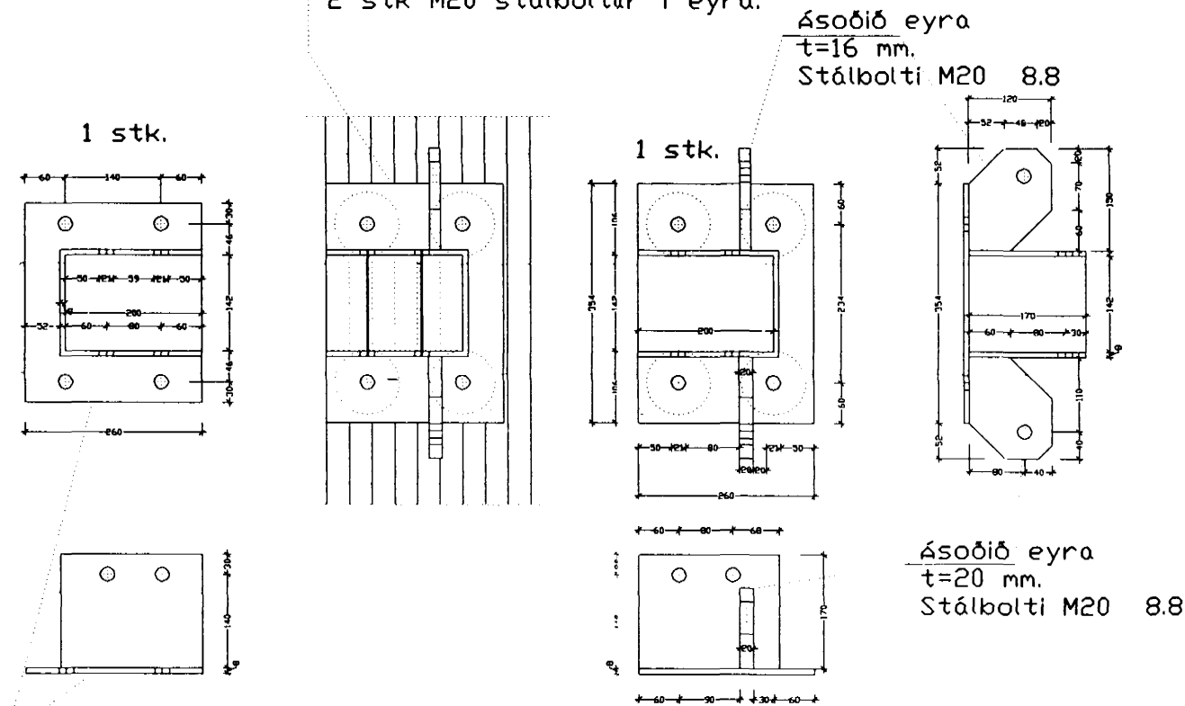
Stálfesting á móti VSV.4. (sama súla) Langband í vegg. 1 samsetning. 2 stk. stálboltar M20 í langband, lengd=200 mm
