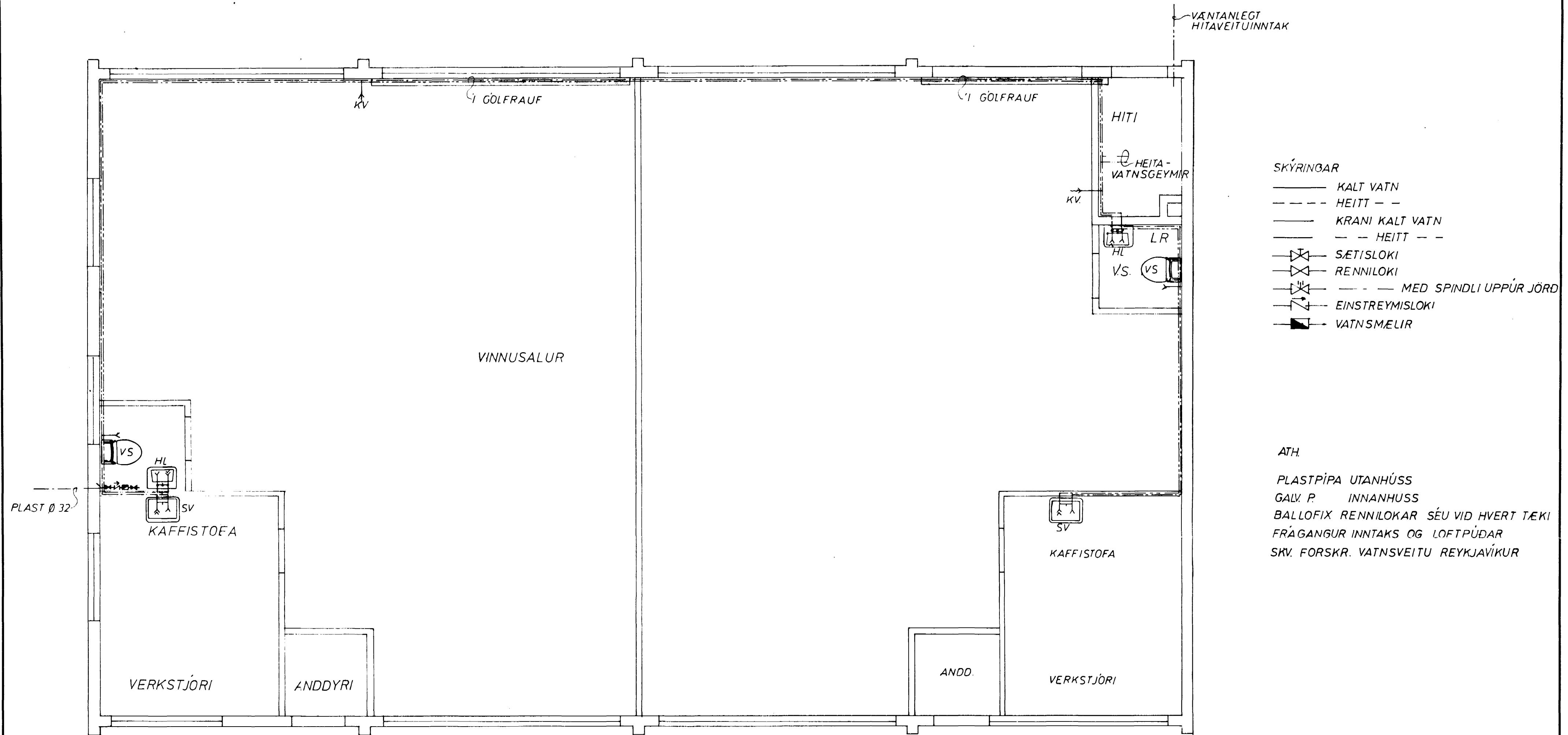
GRUNNMYND 1:50
