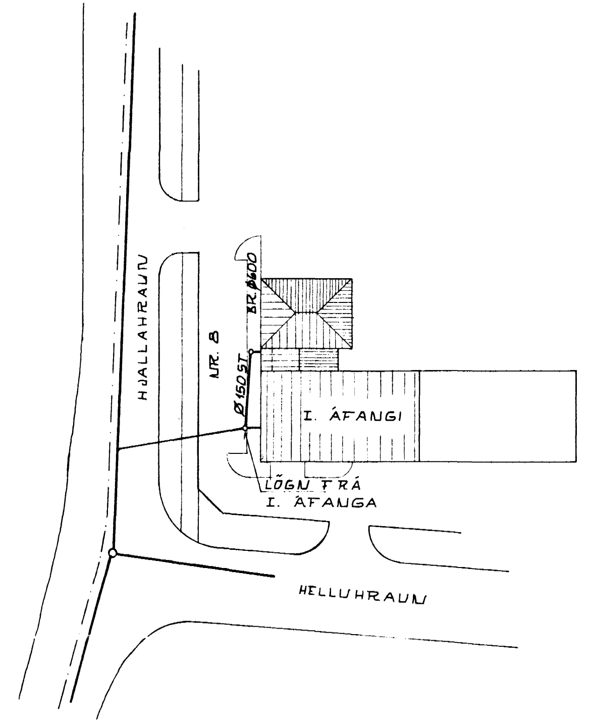
AFSTÖÐUMYND 1:500
