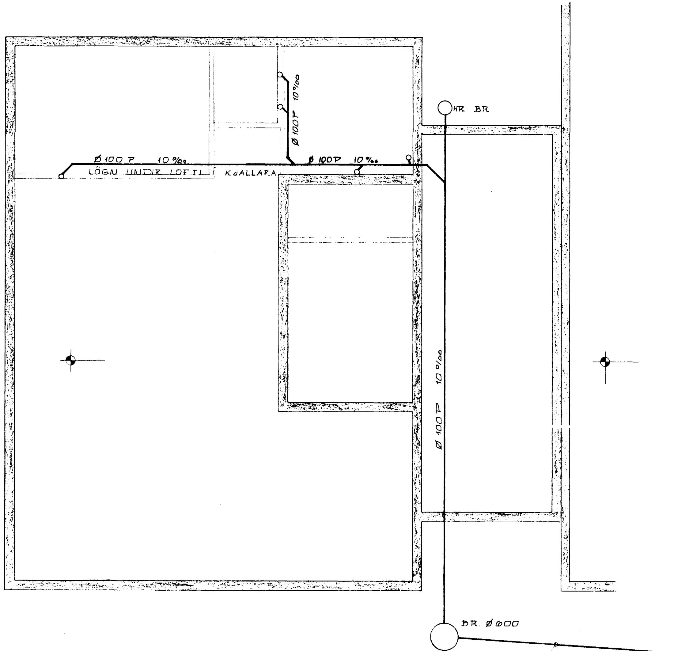
GRUNNMYND 1:50
