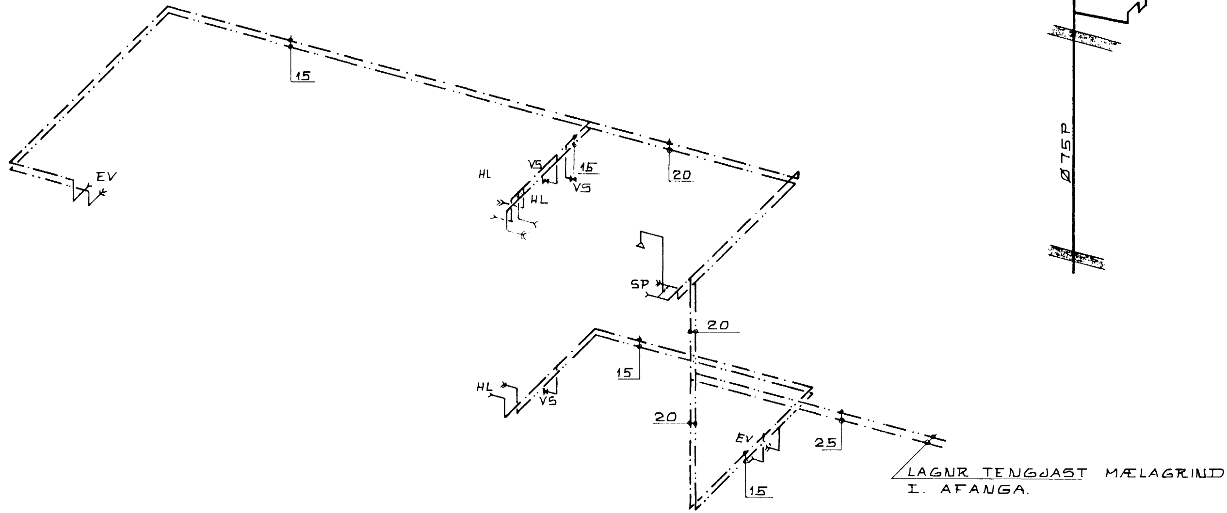
FALLPÍPUR 1:50
