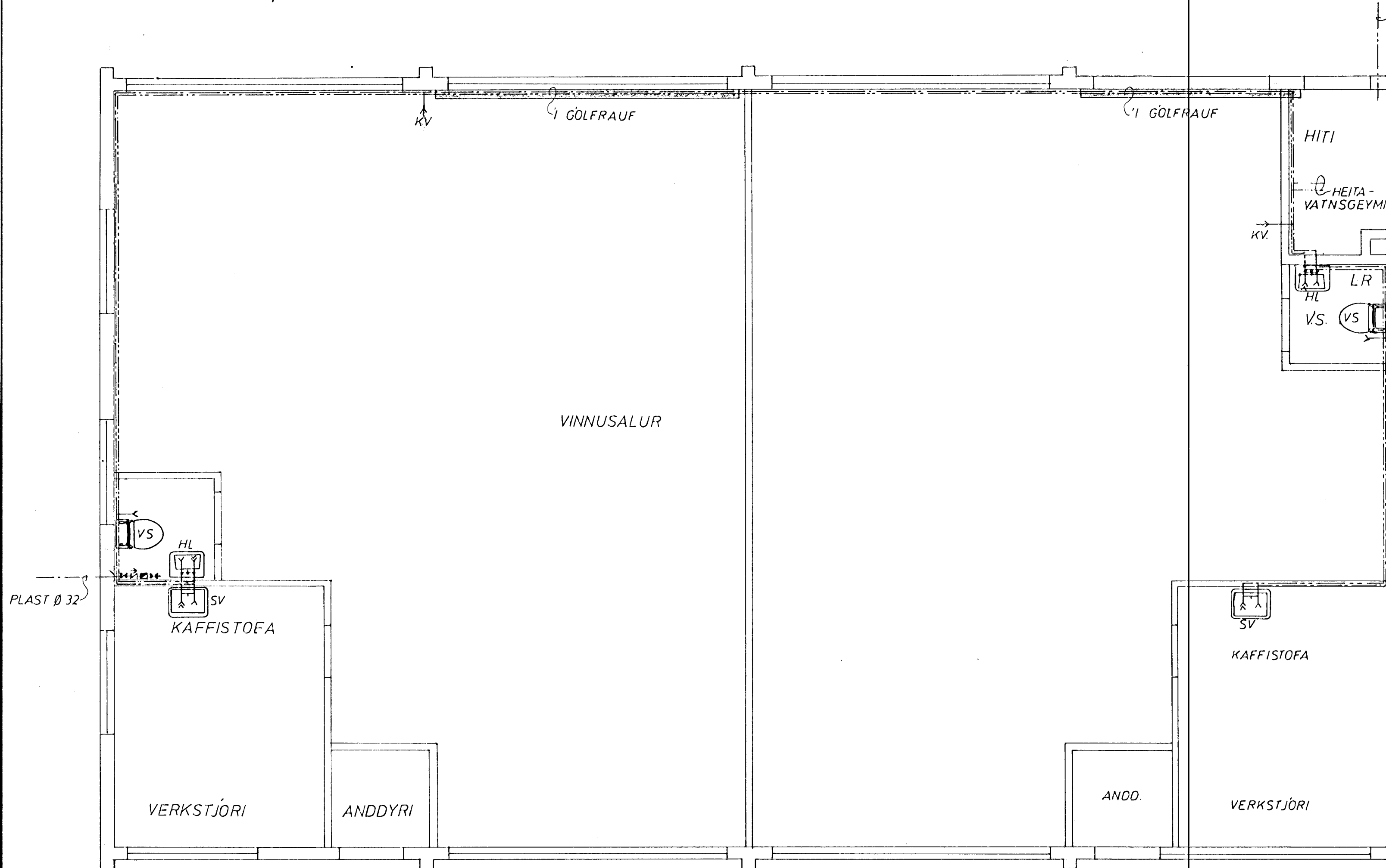
GRUNNMYND 1:50
