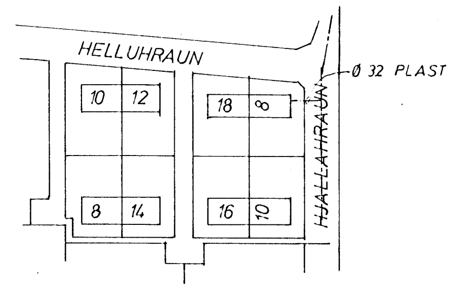
AFSTADA 1:2000
